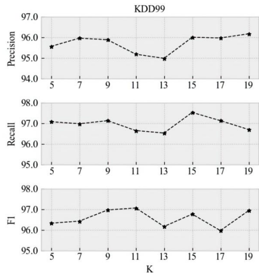
图 5 KDDCUP99 数据集参数敏感性实验
