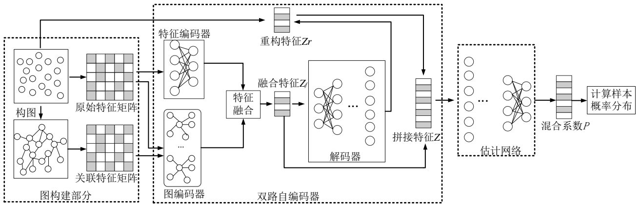
图 3 模型框架
