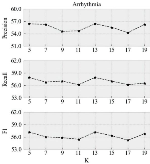
图6 Arrhythmia 数据集参数敏感性实验
