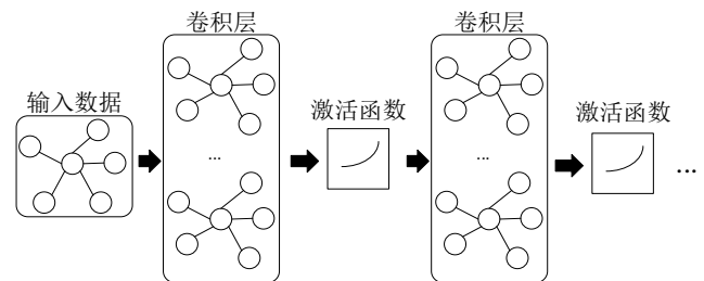
图2 图卷积神经网络基本模型
