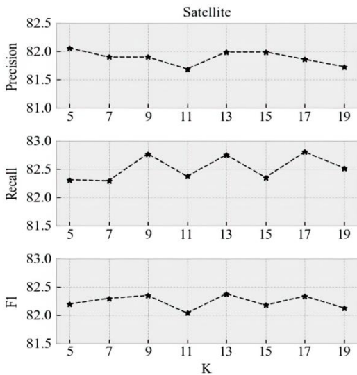
图7 Satellite 数据集参数敏感性实验
