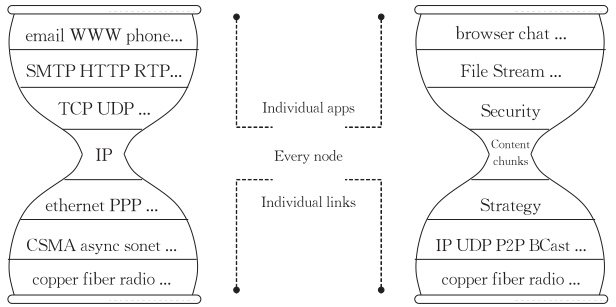
图 4 NDN/CCN 层次结构 [27]
