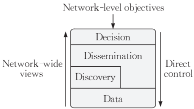
图 5 4D 网络体系结构 [34]
