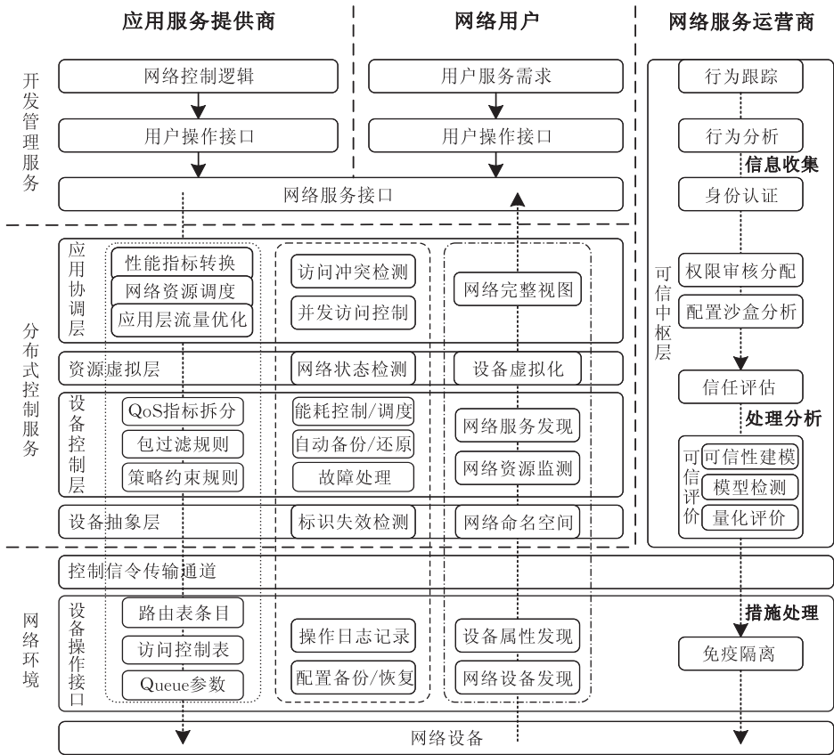
图 12 AFIF 体系框架
