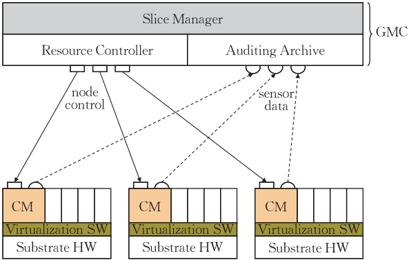
图 7 GMC 资源垂直分片管理 ①
