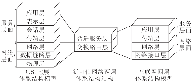
图 10 一体化可信网络 [38]
