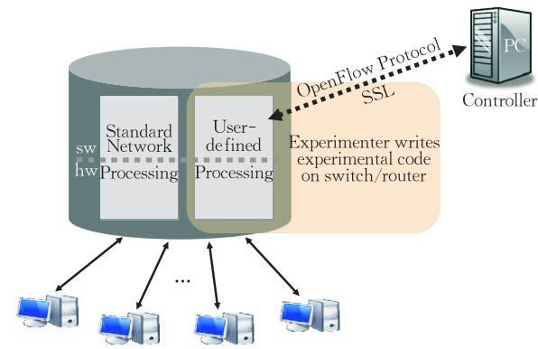
图 2 OpenFlow 体系结构 [19]
