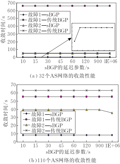
图 4 不同延迟参数 \tau 对 BGP 收敛性能的影响
