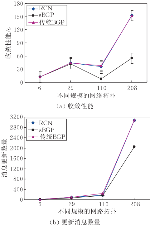
图 6 互联网拓扑的 BGP 性能比较
