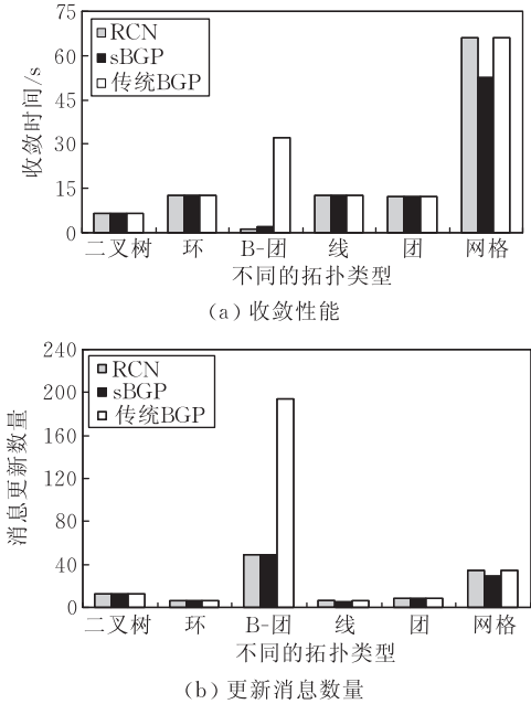
图 5 简单拓扑的 BGP 性能比较
