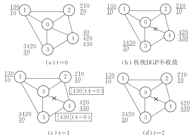
图 3 传统 BGP 和 sBGP 的收敛示意图
