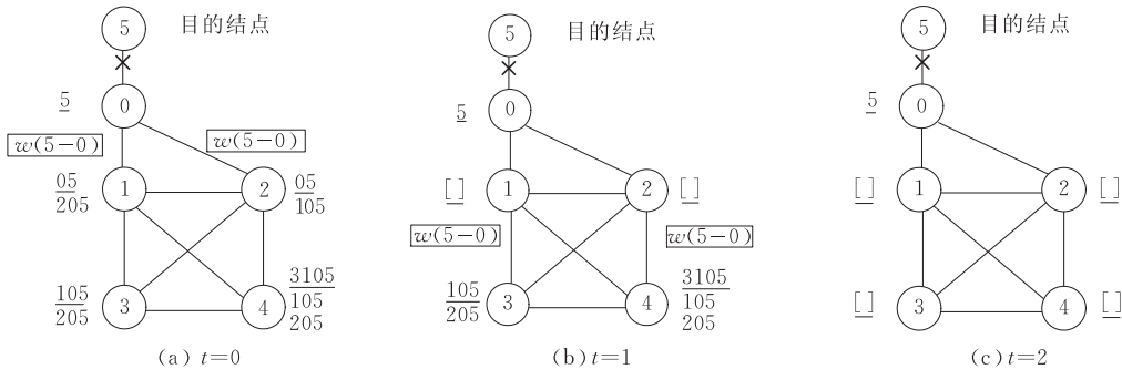
图 2 sBGP 在 B-团拓扑中的收敛过程
