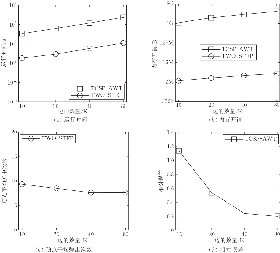
图 6 边的数量对算法性能的影响
