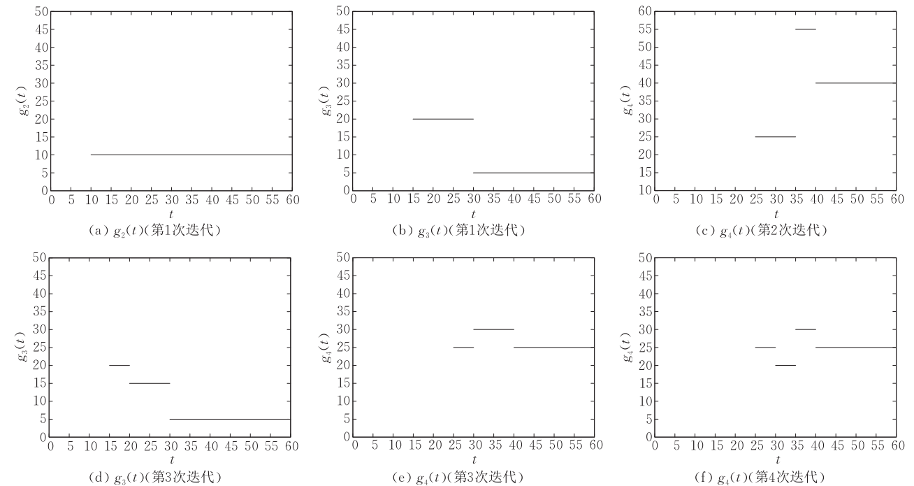
图 4 图 1 例中到达时间-最小代价函数更新过程
