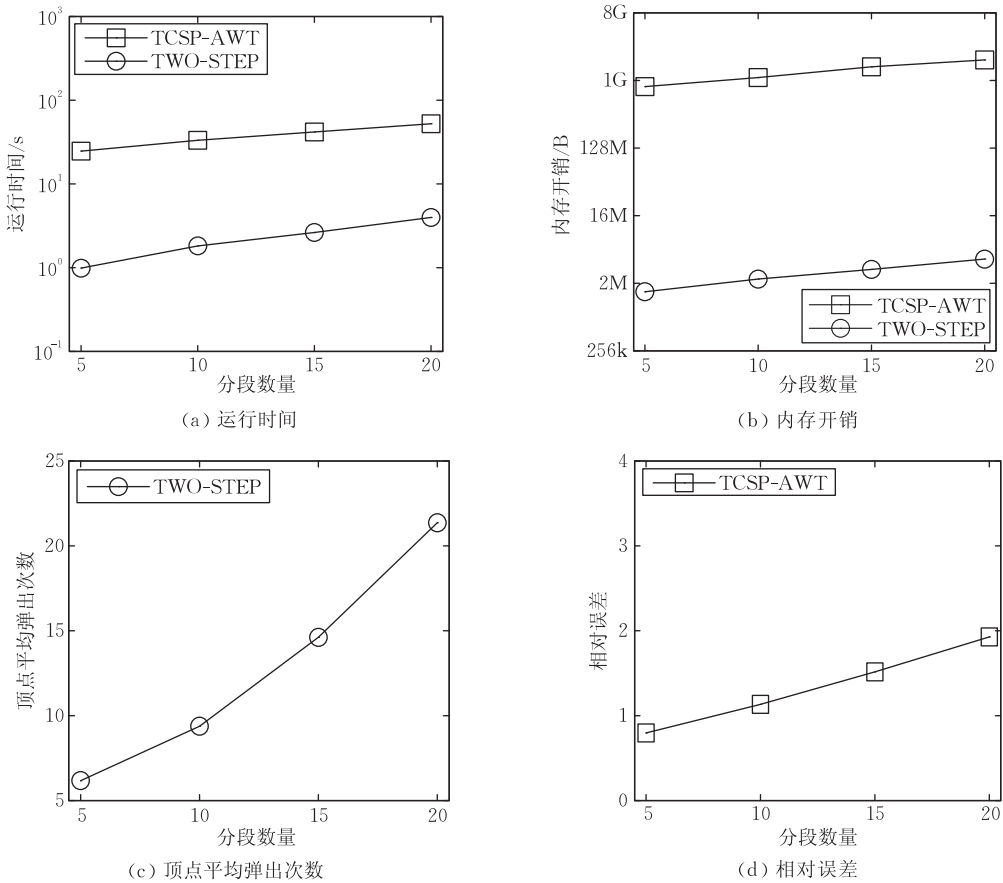
图 9 费用代价函数分段数量对算法性能的影响
