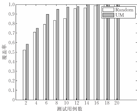
图 4 两种测试策略下的用例数量对比
