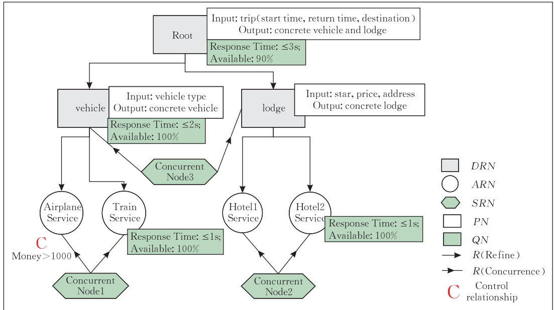
图 1 行程安排服务用户需求模型图例
