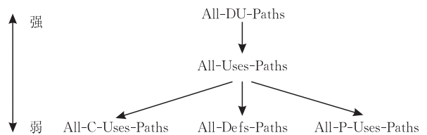
图 2 数据流测试覆盖策略关系
