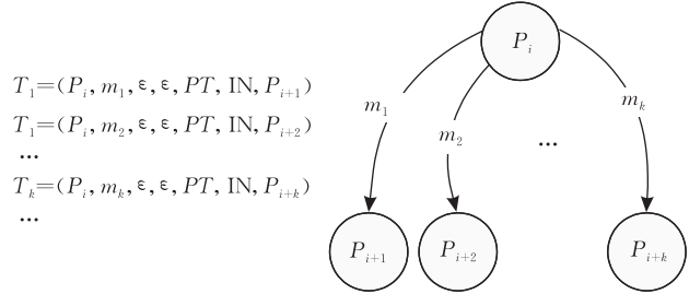
图 5 <pick>活动状态迁移示意图
