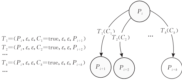
图 4 <switch>活动状态迁移示意图
