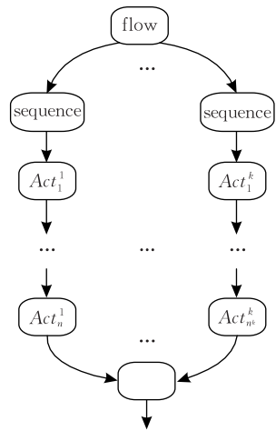
图 10 \langle flow \rangle 中嵌套 \langle sequence \rangle
