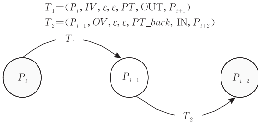
图 3 同步 \langle invoke \rangle 活动状态迁移示意图
