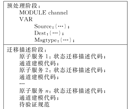
图 12 MCTK 代码的组成
