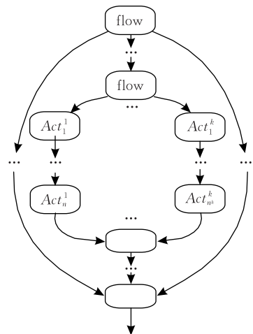
图 11 \langle flow \rangle 中嵌套 \langle flow \rangle
