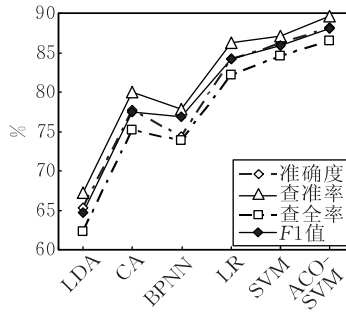
(g) MW1数据集预测结果
