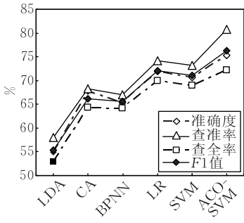
(i) PC2数据集预测结果
