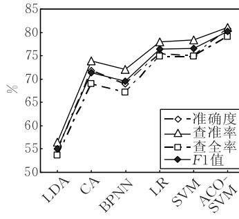
(j) PC3数据集预测结果
