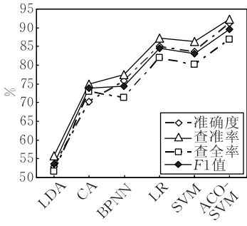
(c) KC3数据集预测结果
