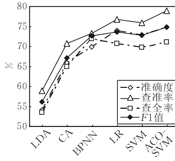
(d) KC4数据集预测结果
