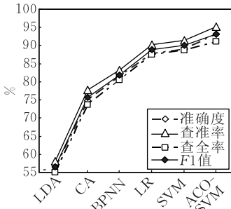
(a) JM1数据集预测结果
