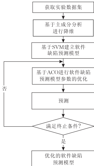
图 1 建立软件缺陷预测模型的流程
