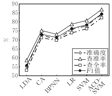
(h) PC1数据集预测结果
