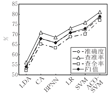
(k) PC4数据集预测结果
