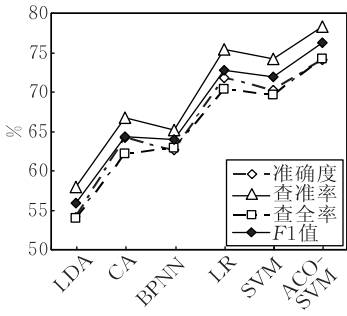
(f) MC2数据集预测结果
