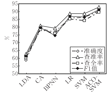
(e) MC1数据集预测结果
