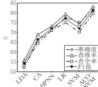
(b) KC1数据集预测结果
