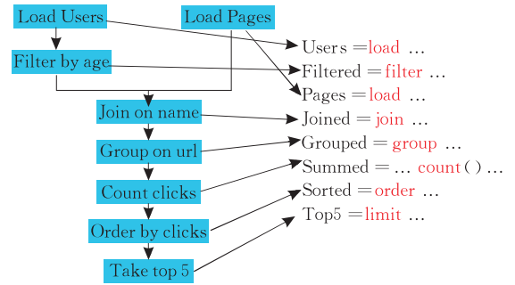
图 3 Pig Latin 的一个查询示例(右边为实际脚本)
