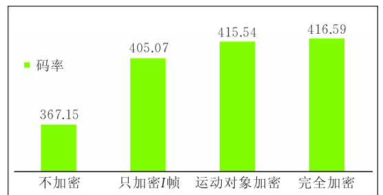
图 12 运动对象加密与其它加密算法码率比较图
