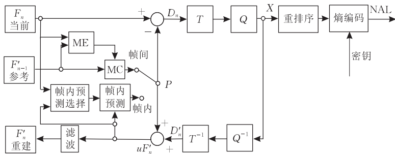
图 1 编码端加密流程图
