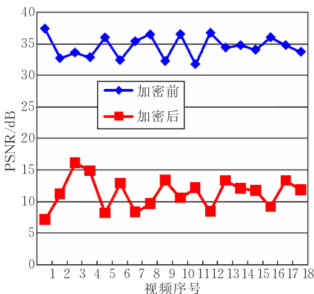
图 11 加密前后 PSNR 值比较图
