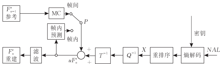
图 2 解码端解密流程图
