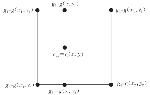
图 1 同类块 B 的示意图
