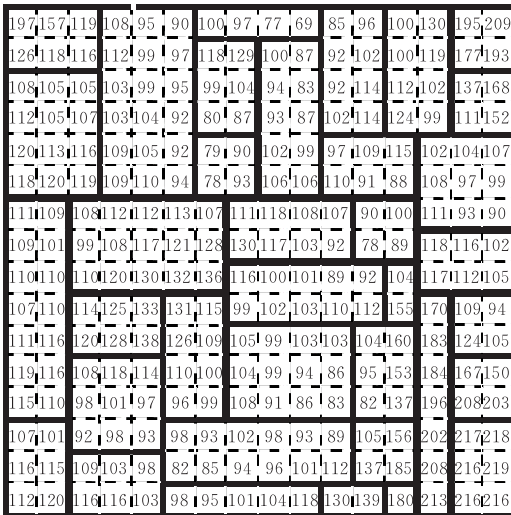
(a) RNAMC 方法分割后的同类块
