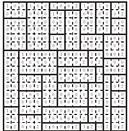
(b) (a) 对应的 R 矩阵
