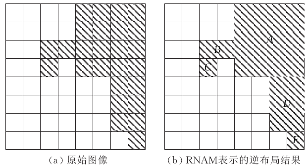
图3 RNAM表示的一个简单例子
