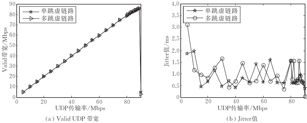
图 11 基于 CERNET2 的 VegaNet 中带宽和 Jitter 值测量
