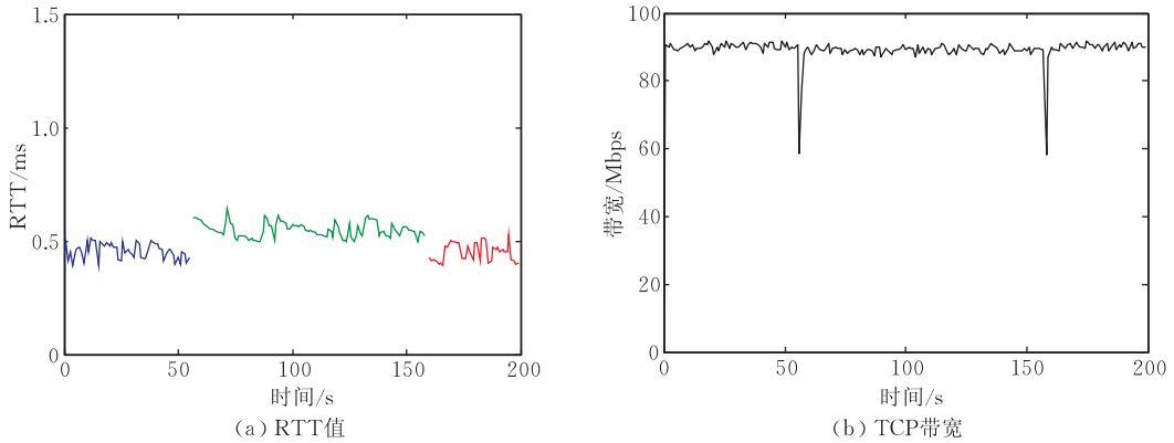
图 14 实验室环境 VegaNet 中 RTT 和 TCP 带宽测量
