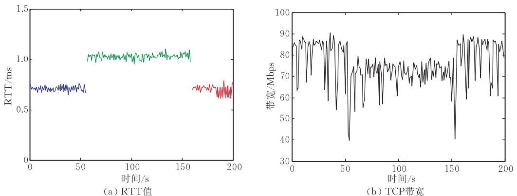
图 13 基于 CERNET2 的 VegaNet 中 RTT 和 TCP 带宽测量
