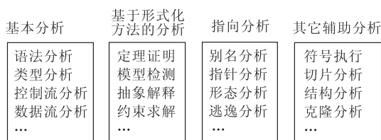
图 2 主要的静态分析技术
