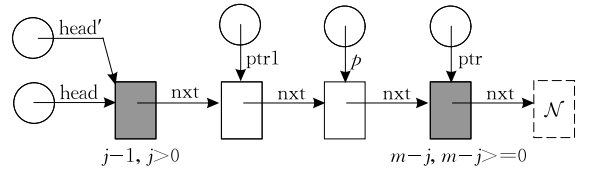
图 18 return 语句前形状图的一种情况
