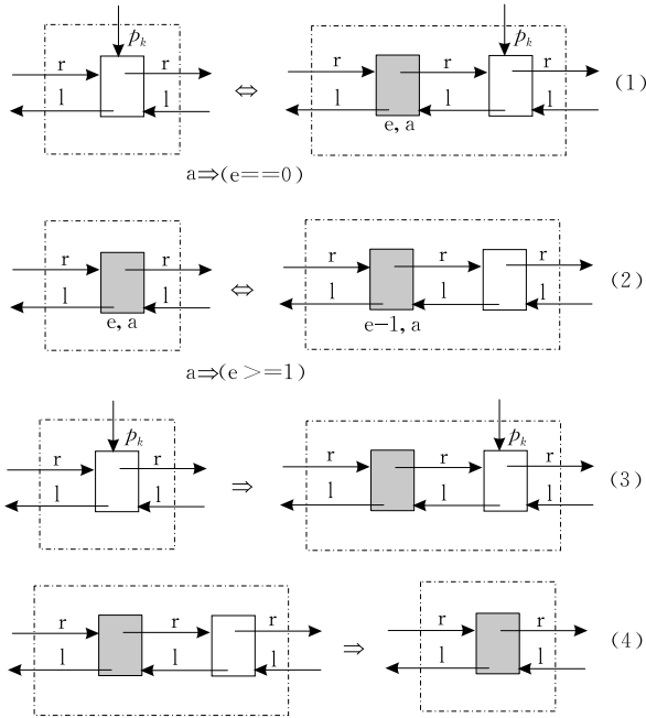
图 5 从等价规则得到的蕴涵规则
