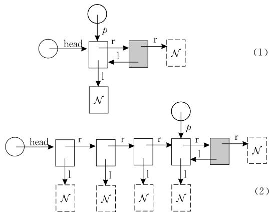
图 15 循环不变形状图推断过程报告错误的例子
