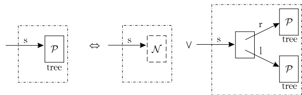
图 11 从二叉树定义得到的等价规则
