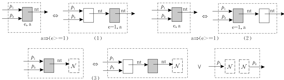
图 3 (循环)单链表的等价规则的 3 个例子
