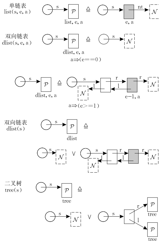
图 2 形状谓词定义的一些例子
