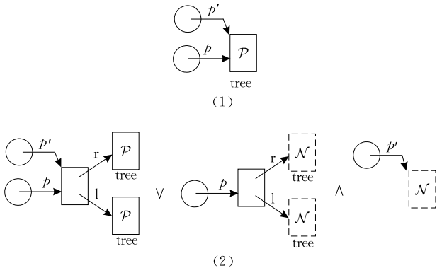
图 19 二叉排序树插入函数的前后形状图
