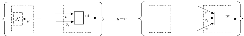
图 6 指针赋值语句的一条规则
