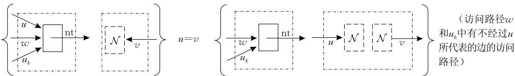
图 7 指针赋值语句的另一条规则
