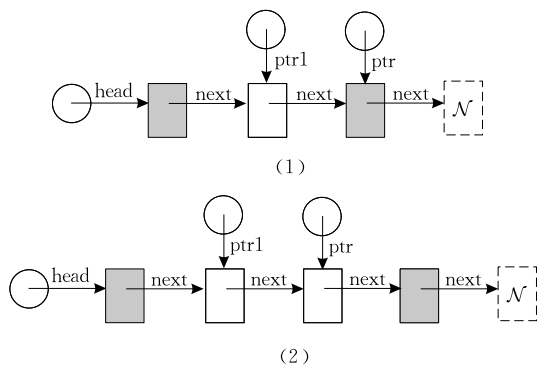
图 8 形状图的两个例子
