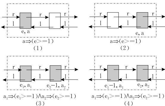
图 10 临界对的两个例子
