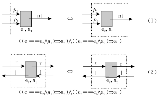
图 4 对浓缩节点的约束数据进行变换的部分等价规则
