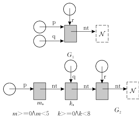
图 12 帮助理解定义 5 的两个形状图
