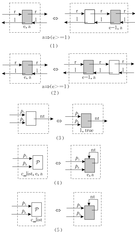
图 9 等价规则的一些例子
