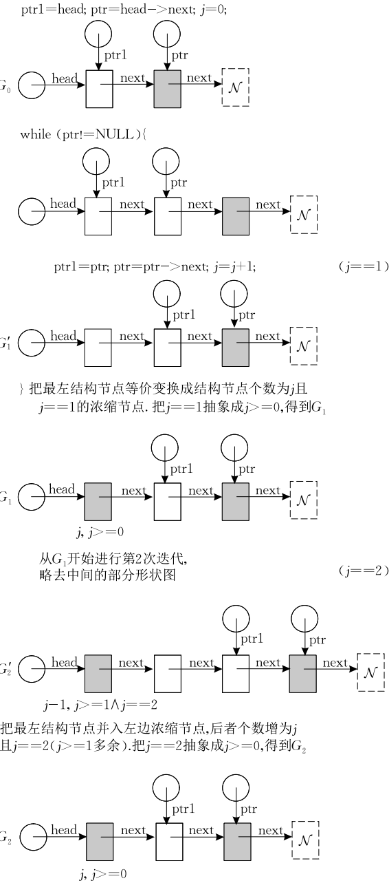
图 14 推断循环不变式的迭代过程
