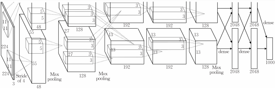
图 3 AlexNet 模型结构 [6]
