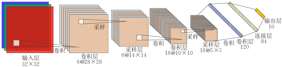
图 2 卷积神经网络的典型结构 [12]
