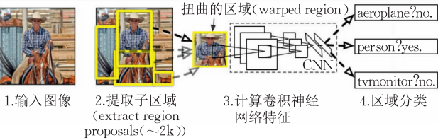
图 13 R-CNN 目标检测算法的流程图 [44]
