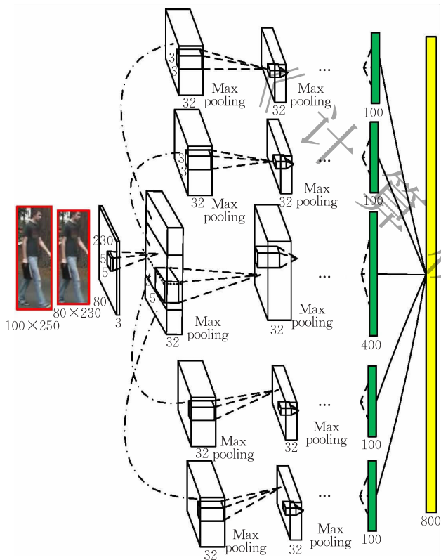
图 24 Cheng 等人提出的多通道 Deep CNN 网络结构 [101]
