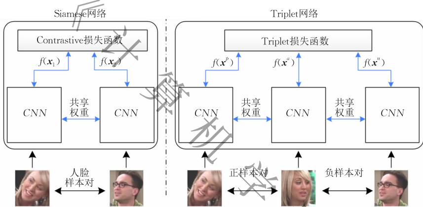
图 12 Siamese 网络和 Triplet 网络的结构示意图(Siamese 网络包含两个架构相同且参数共享的 CNN 模型, 以一对图像作为输入, 使用 contrastive 损失函数进行训练. Triplet 网络包含三个相等的 CNN, 以图像三元组作为输入, 使用的损失函数为 triplet 损失函数)
