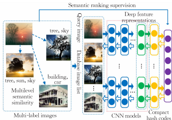
图 27 DSRH 图像检索方法的流程示意图 [144]
