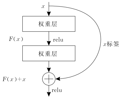
图 6 残差网络的学习模块
