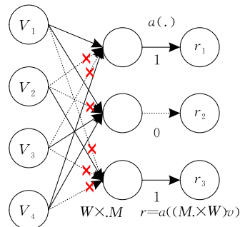
(b) DropConnect 网络示意图
