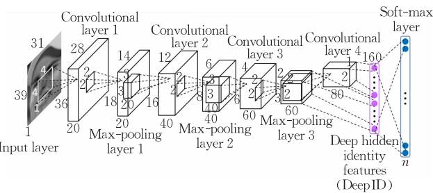
图 23 DeepID 网络结构 [15]
