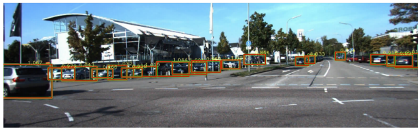
图 15 DenseBox 在 KITTI 数据集的车辆检测结果 [52]
