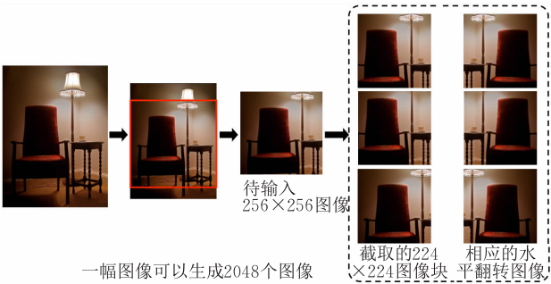
图 8 数据集扩增
