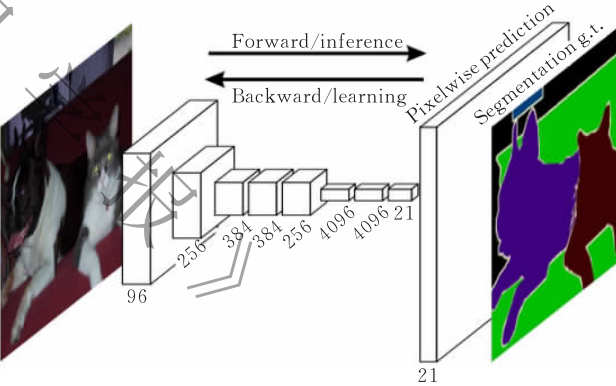
图 16 全卷积网络的结构示意图 [66]
