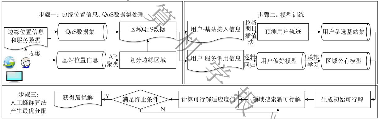
图 2 MECFLD_QoS 方法图
