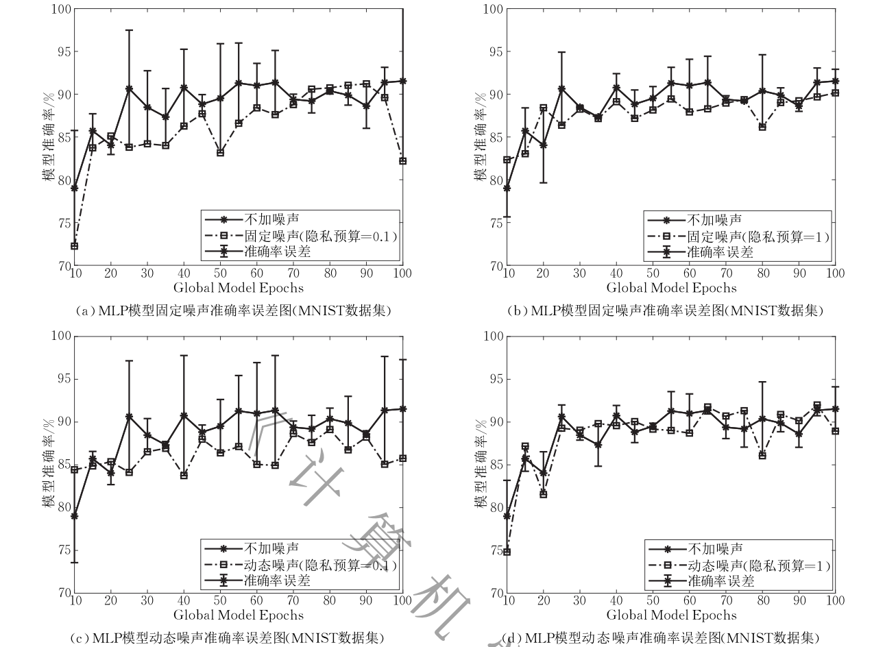
图 4 不同隐私保护方案在设置不同的初始隐私预算情况下对模型准确率的误差影响
