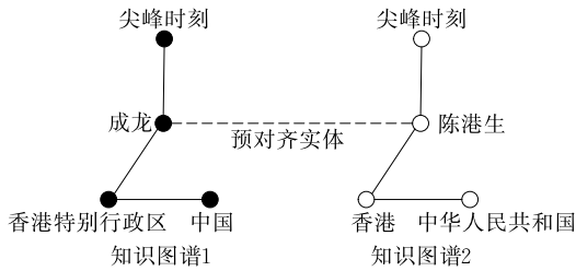
图1 实体对齐任务示意图
