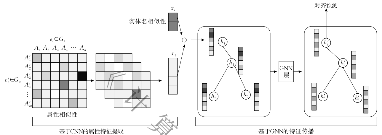
图 16 特征提取和特征传播框架图
