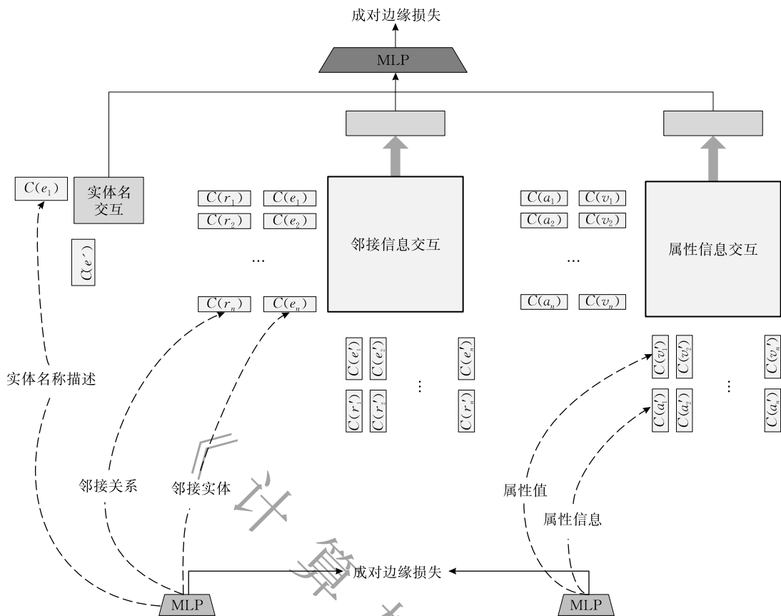
图 18 BERT-INT-2 模型图
