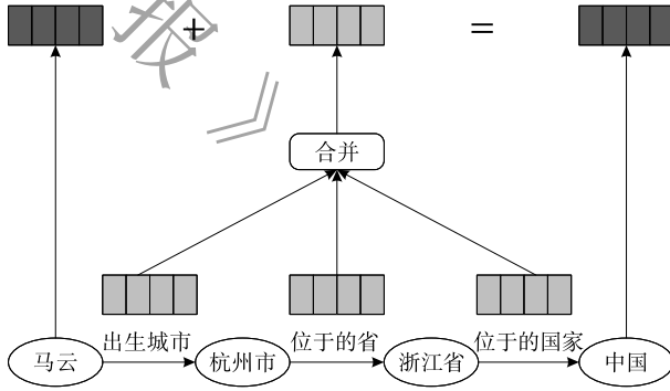
图 7 PTransE 模型
