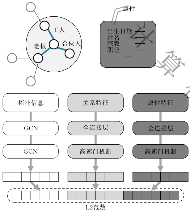
图 14 HMAN 模型图
