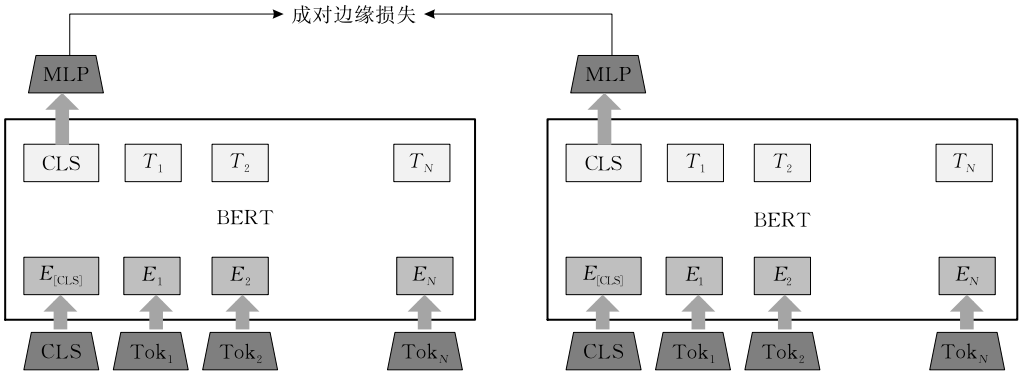
图 17 BERT-INT-1 模型图
