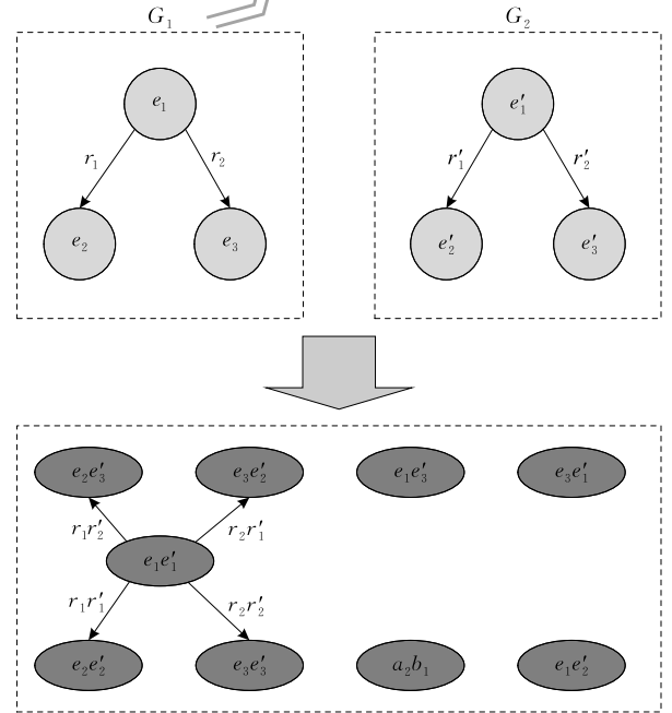
图 15 成对连接图(PCG)
