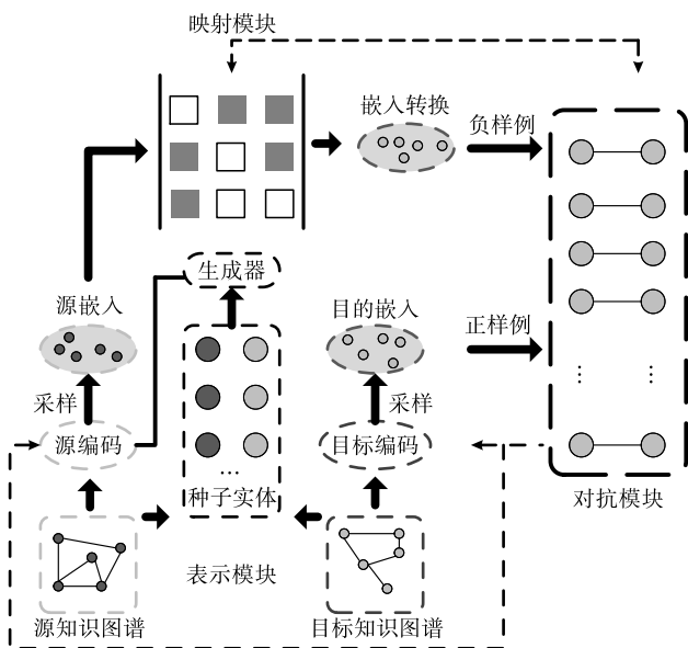
图 8 AKE 模型
