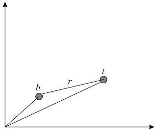
图 5 TransE 模型
