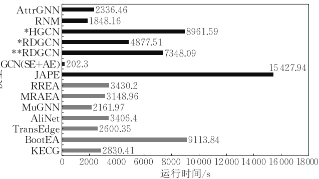
图 19 不同模型在同一数据集 DBP15K ZH-EN 上运行时间对比
