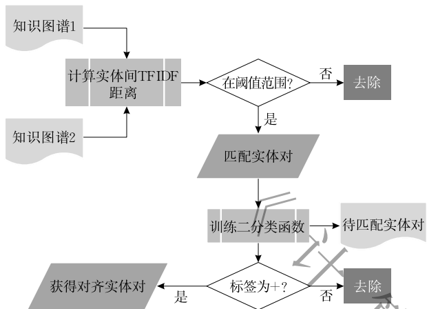
图 2 TFIDF 实体对齐示意图
