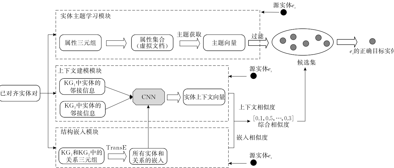
图 11 CTEA 方法框架
