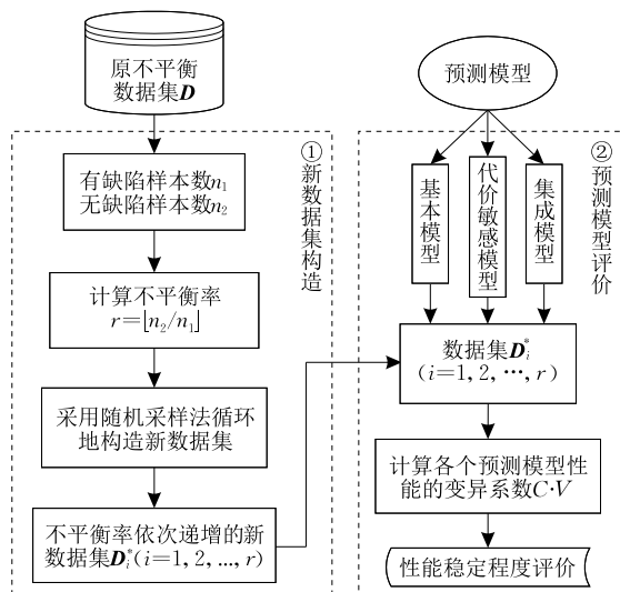
图1 方法流程
