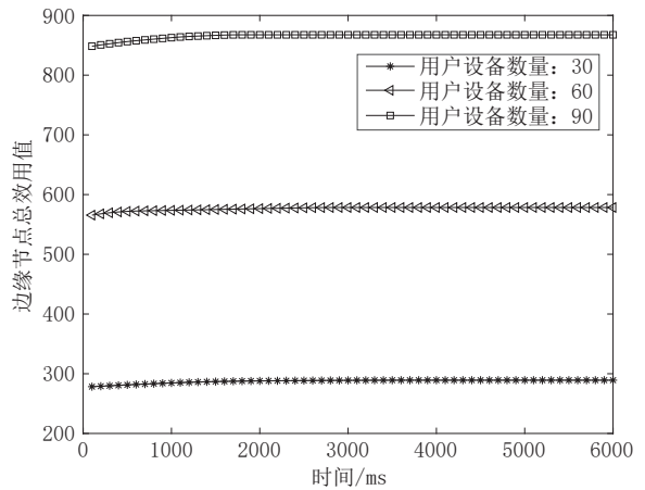
图12 不同用户设备数量边缘节点总效用值
