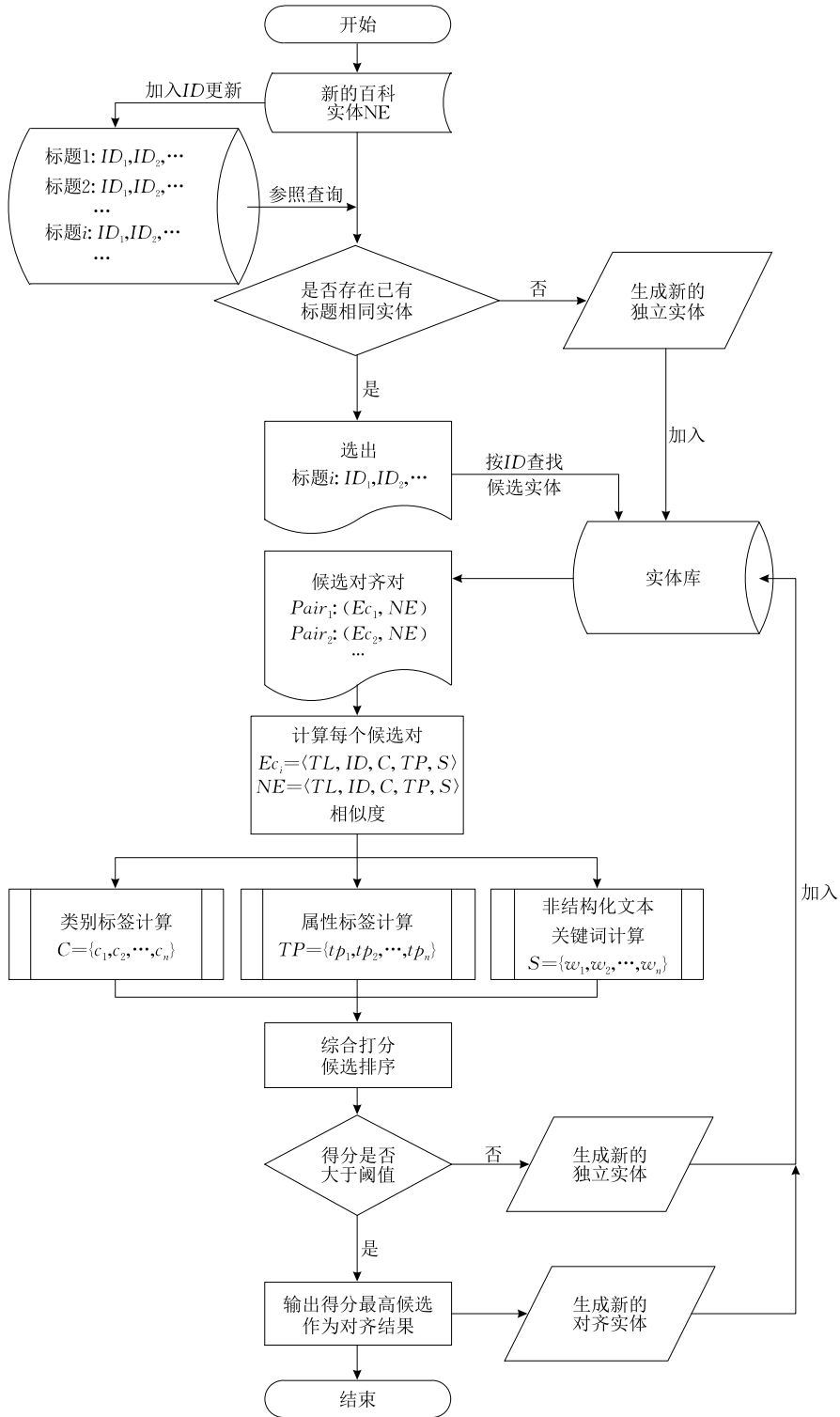
图 1 算法流程图
