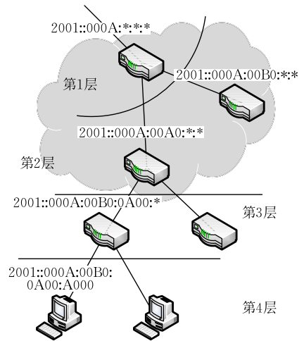
图 6 分层地址动态机制
