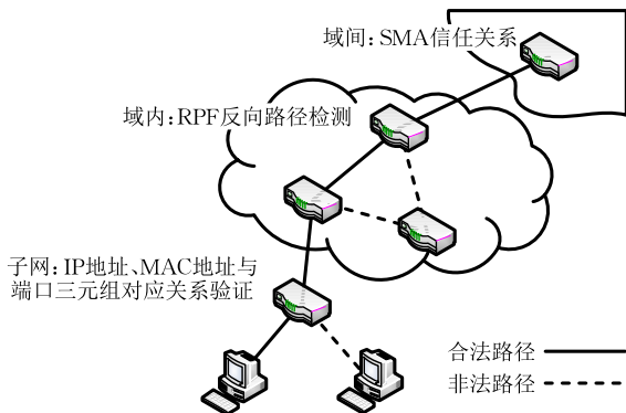
图 2 SAVA 三层源地址验证架构示意
