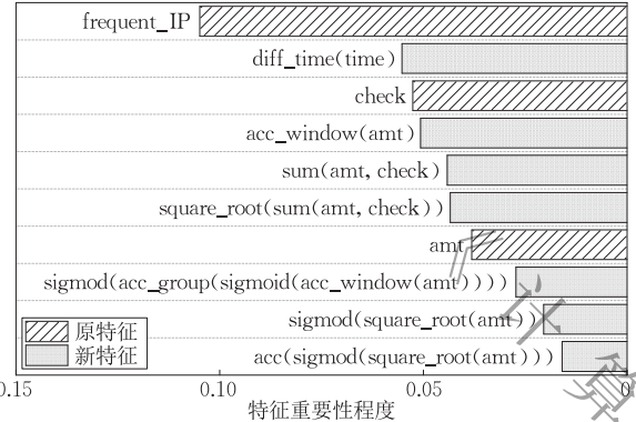
图 12 数据集 2 上实验设置 2 的重要性前 10 的特征
