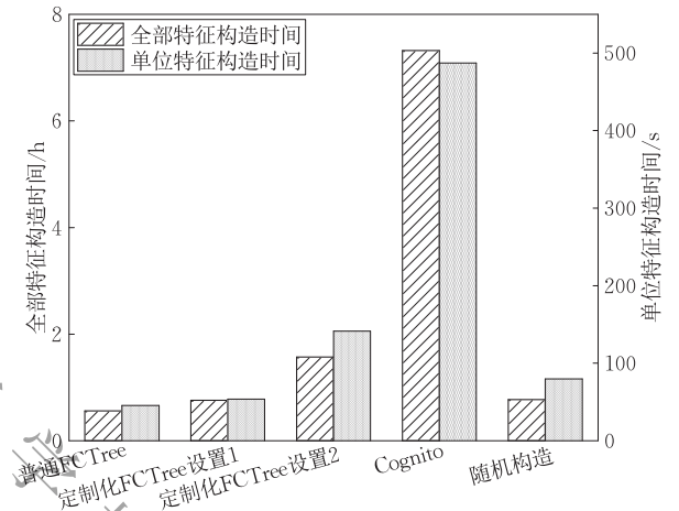
图 15 银行 B2C 线上支付数据集特征构造耗时
