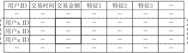
图 5 时间窗口方式的转换函数的作用域
