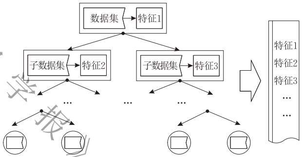
图 6 特征构造树结构
