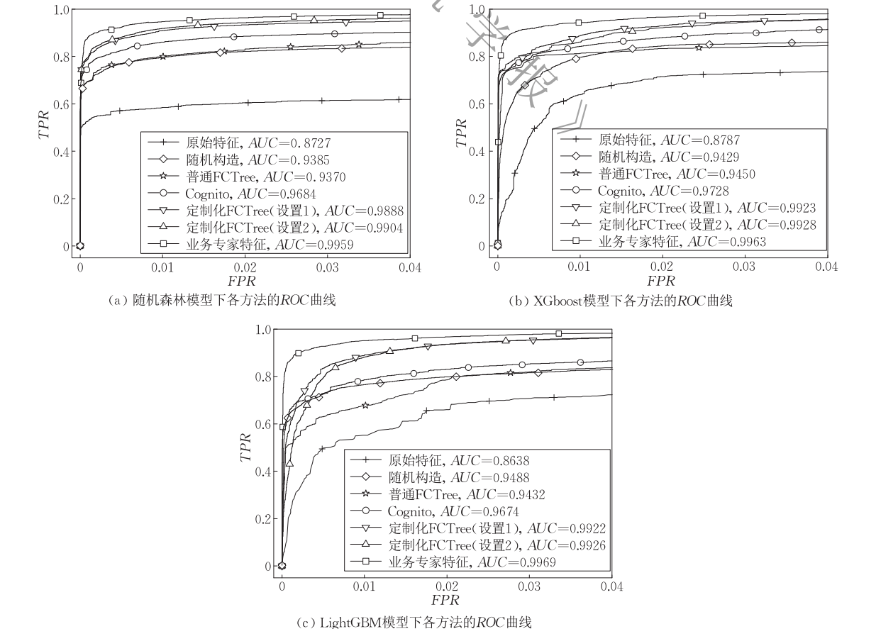
图 13 银行 B2C 网络支付数据集上不同方法构造的特征在各模型的 ROC 表现
