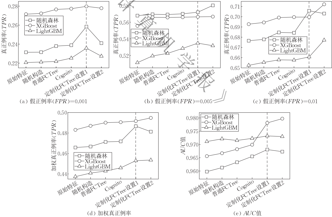
图 10 第三方移动支付数据集上不同特征构造方法下的模型性能对比
