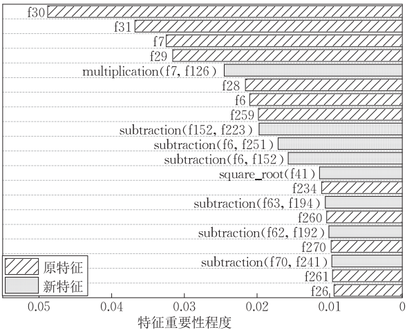
图 8 数据集 1 上实验设置 1 的重要性前 20 的特征
