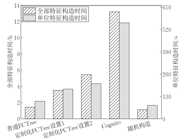
图 14 第三方移动支付数据集特征构造耗时
