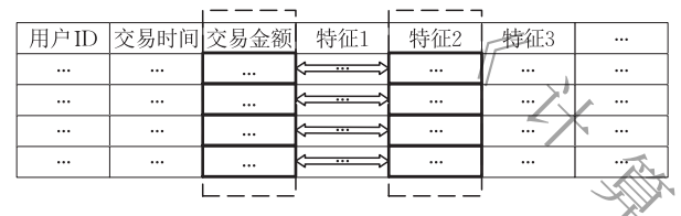
图 3 纵向方式的转换函数的作用域
