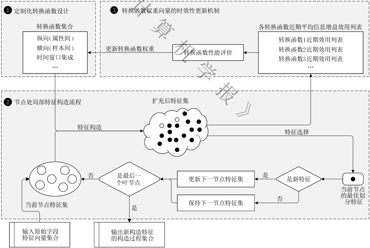
图 2 特征构造树算法整体框架
