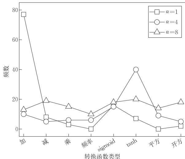
图 7 不同 \alpha 取值下转换函数的频数分布
