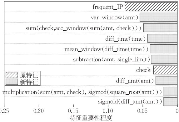
图 11 数据集 2 上实验设置 1 的重要性前 10 的特征
