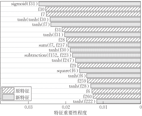
图 9 数据集 1 上实验设置 2 的重要性前 20 的特征
