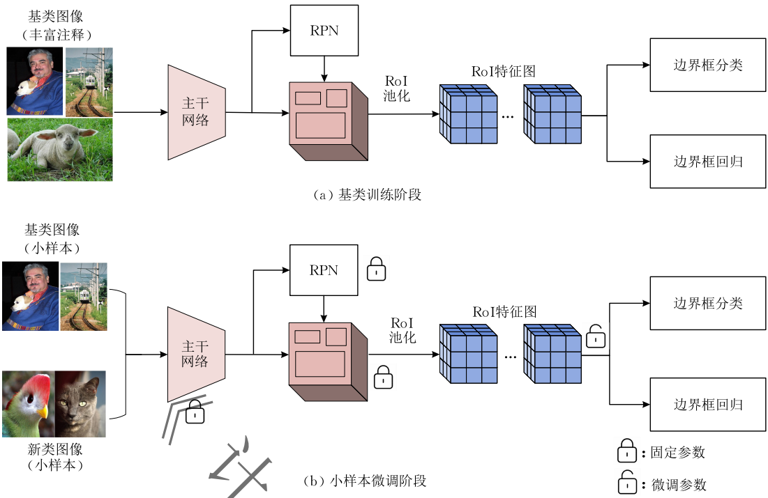
图 6 基于迁移学习的两阶段小样本检测框架
