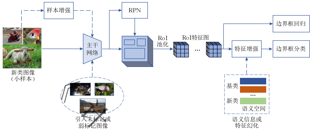
图 7 基于数据增强的小样本检测方法
