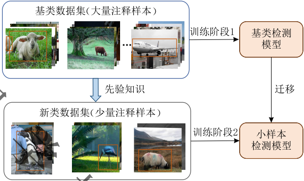
图 2 小样本目标检测示意图
