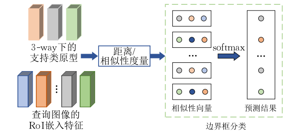
图 9 边界框分类的度量模块实现
