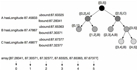
图 5 基于数字的线段树的实例
