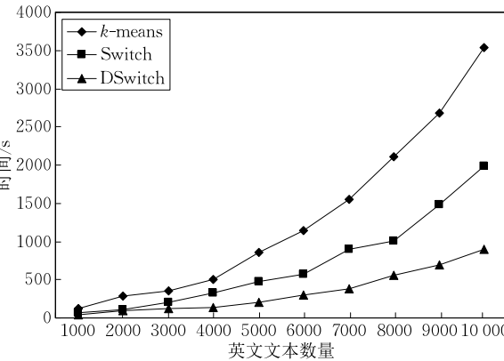
图 8 不同算法英文文本聚类时间对比
