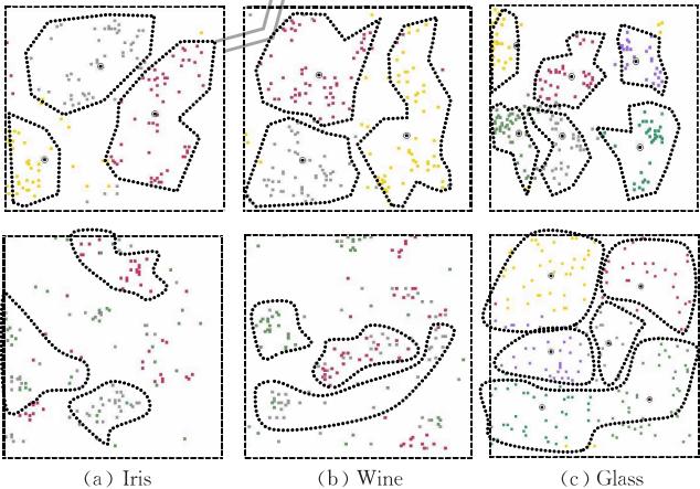
图 10 DSwitch 和 Switch 算法聚类效果对比图
