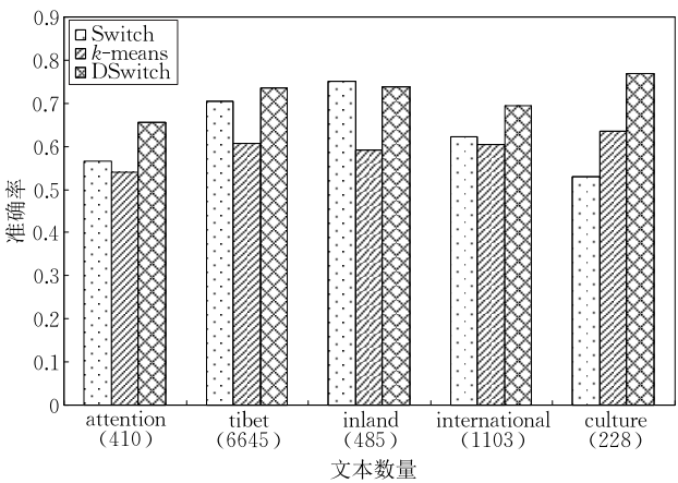
图 6 不同算法 Web 文本聚类的准确率 P 比较
