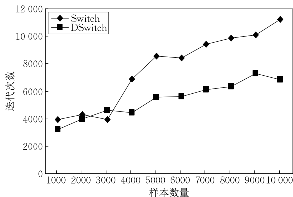
图 11 DSwitch 和 Switch 算法迭代次数比较
