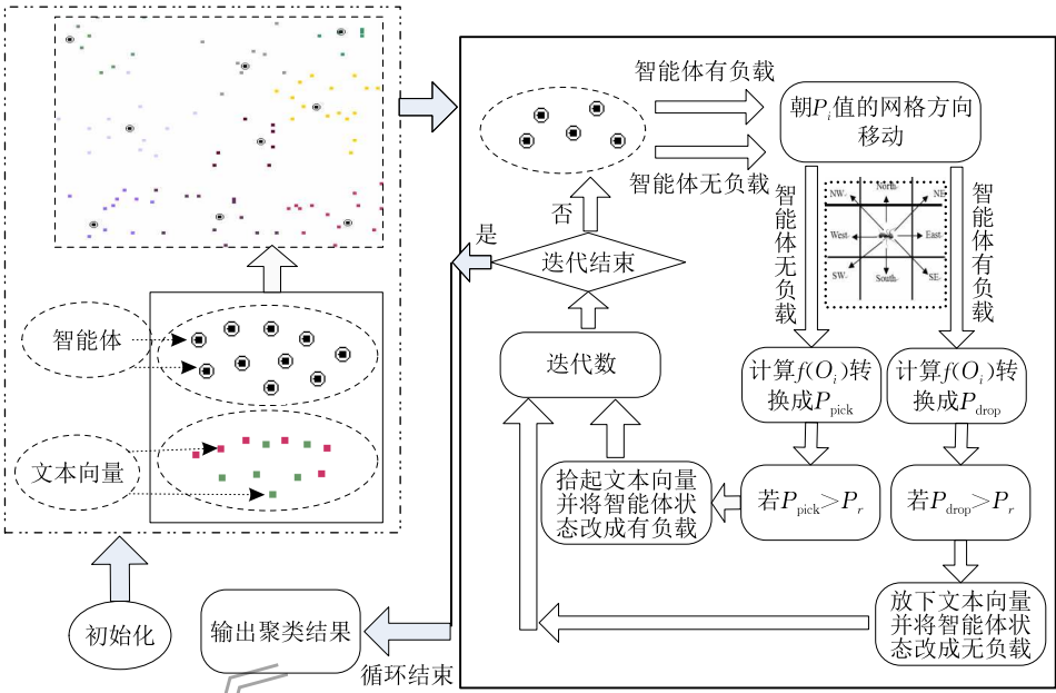
图 1 基于智能体的 Web 文本聚类方法内部原理图
