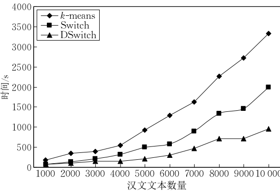
图 9 不同算法汉文文本聚类时间对比
