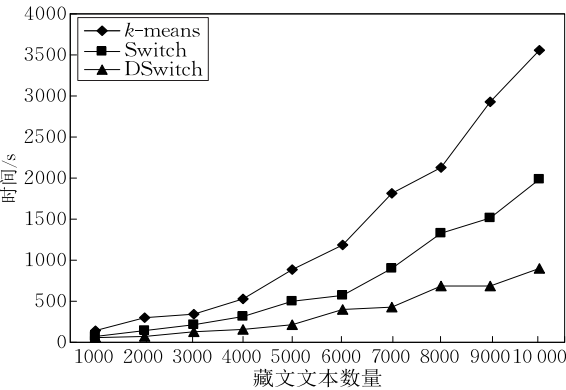
图 7 不同算法藏文文本聚类时间对比
