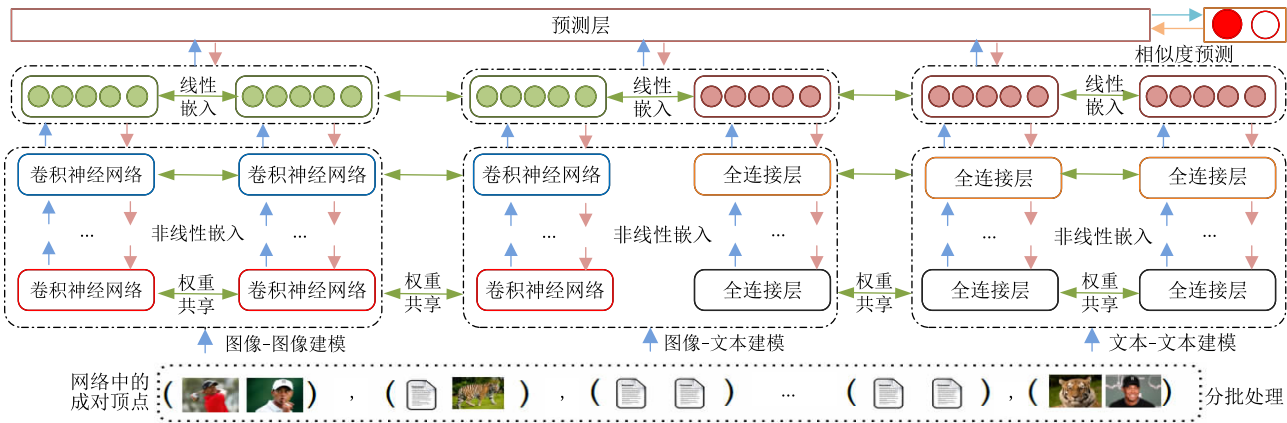
图 9 HNE 模型架构
