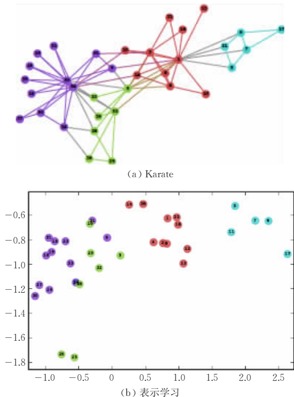
图 1 网络表示学习示例图
