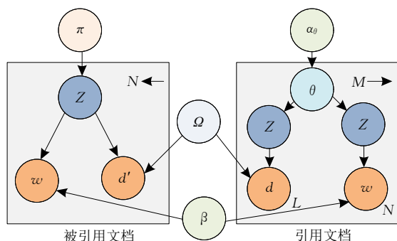
图 7 Link-PLSA-LDA 模型
