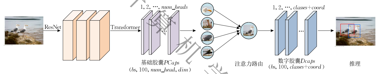
图 2 CIRA_DETR 模型中基于胶囊推理模块的目标检测实现原理
