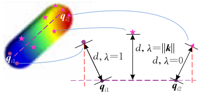
图 4 特征点与香肠区域之间的距离示意图(圆圈、三角形和星星分别代表分布在香肠区域不同位置的样本)
