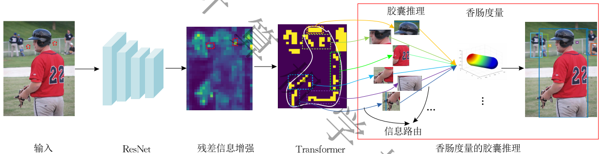
图 1 基于胶囊推理和残差增强的全推理目标检测网络(CIRA_DETR)结构
