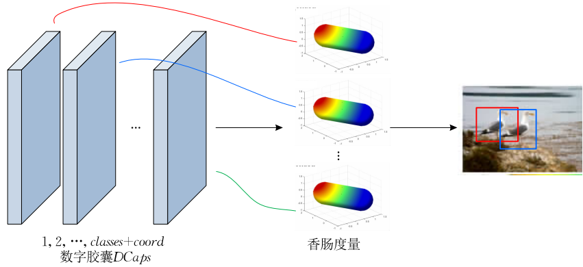
图 3 CIRA_DETR 模型中基于香肠度量的目标检测实现原理
