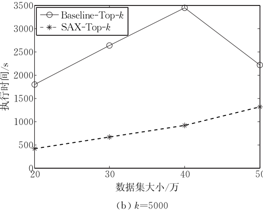
图 8 不同数据集大小对执行时间的影响 (image-960)
