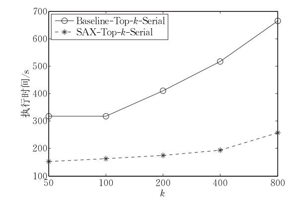
图 6 单机环境下的执行时间对比 (image-128-2w)
