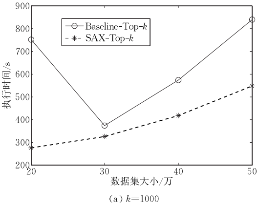
图 7 不同数据集大小对执行时间的影响 (image-128)
