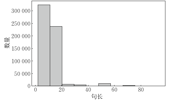
图 5 句子长度分布图
