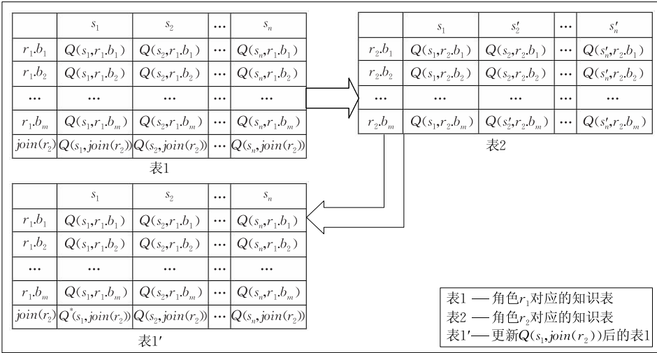
图 9 知识融合示意图
