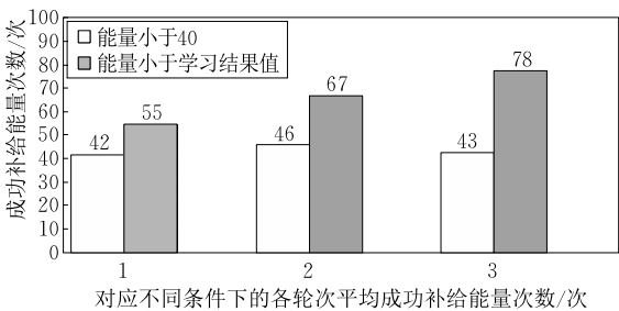
图 12 按照不同的方式角色转换并补给能量成功次数比较
