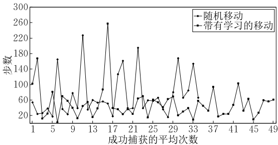
图 11 能量充足条件下机器狗捕获猎物情况
