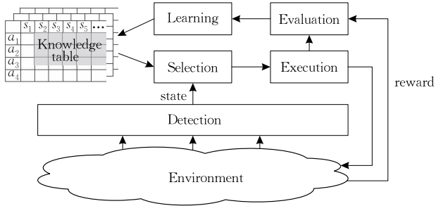
图 4 SA 的自适应学习过程
