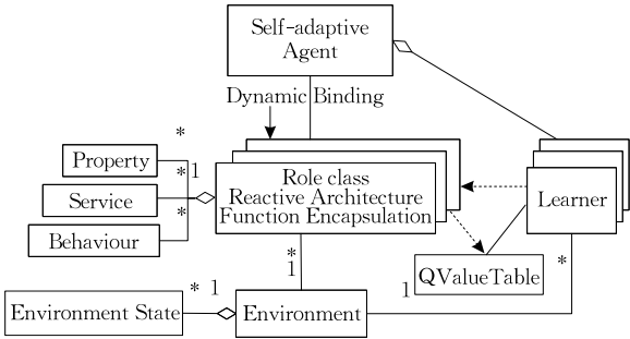
图 6 基于动态绑定自适应机制和强化学习方法的自适应系统构造框架
