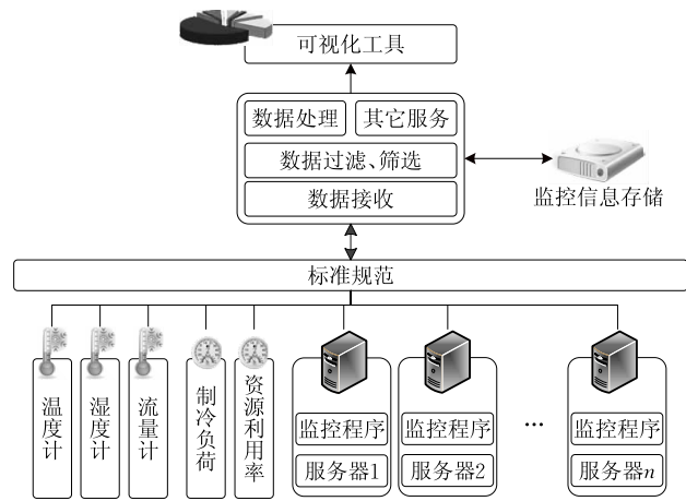
图 2 分布式监控系统框架
