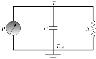
图 4 RC 模型 [30]
