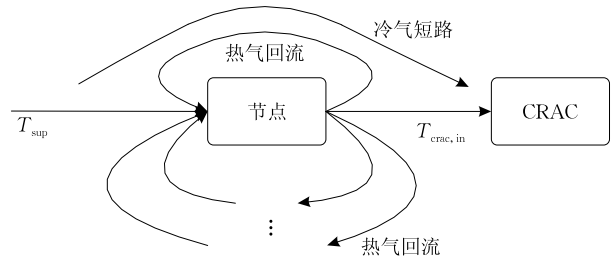
图3 节点交叉热影响模型 [29]
