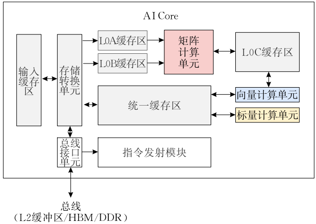
图 1 AI Core 架构示意图
