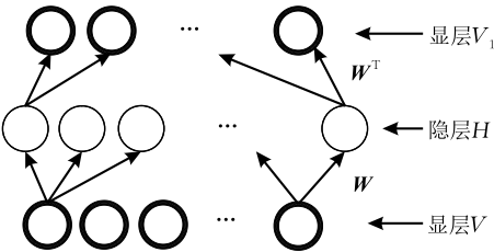
图3 等价RBM图模型
