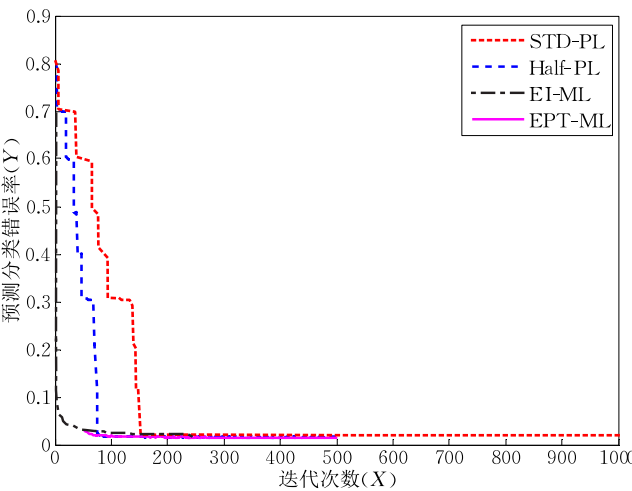
图 16 Mnist 数据集预测分类错误率
