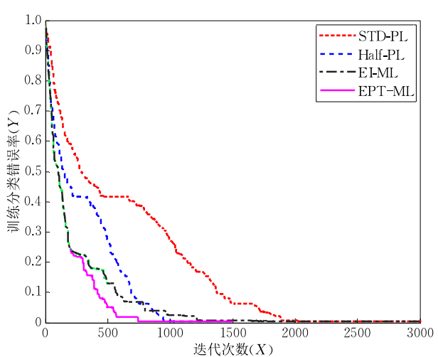
图 11 CMU PIE 数据集训练分类错误率
