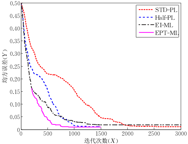
图 10 CMU PIE 数据集均方误差收敛结果
