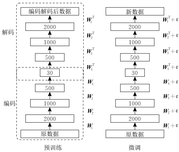
图 5 深度栈式自编码网络数据非线性降维过程
