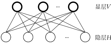
图2 RBM无向图模型
