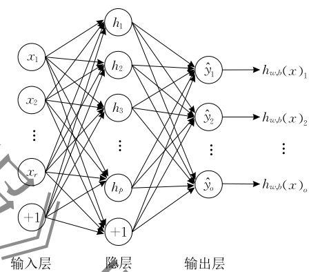
图 1 含有一个隐层和输出层的全连接前馈神经网络
