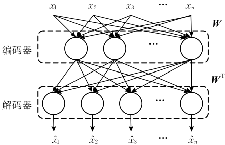
图4 一种Auto-Encoder结构
