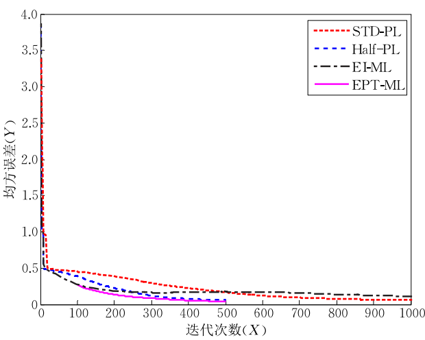
图 18 ORL 数据集均方误差收敛结果
