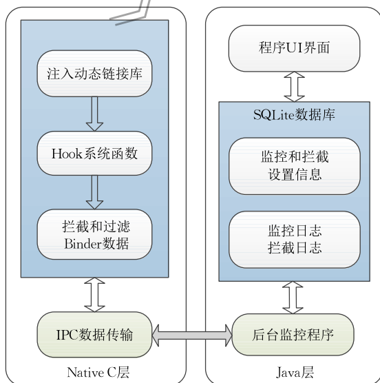
图 3 Android 动态分析架构
