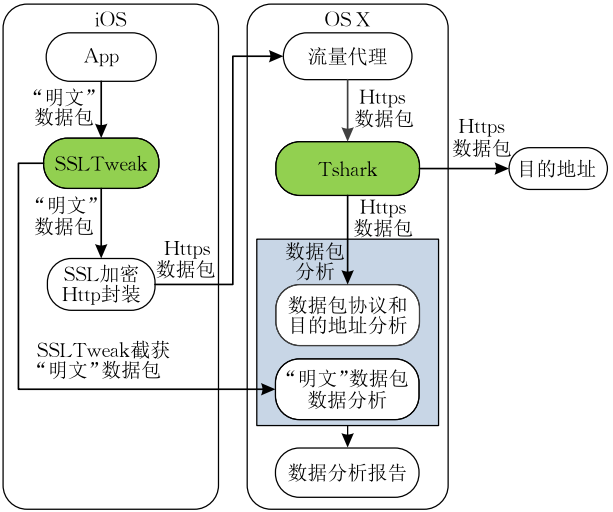
图 6 iOS 系统数据分析框架
