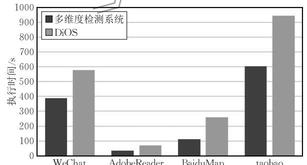
图 11 执行时间对比
