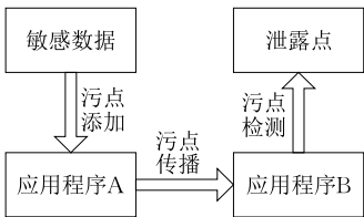
图 4 ExDroid 简化模型
