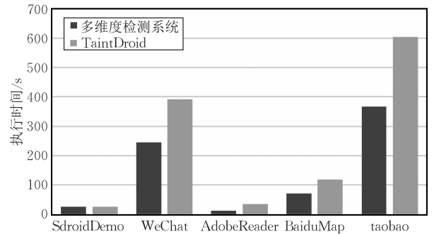
图 9 执行时间对比
