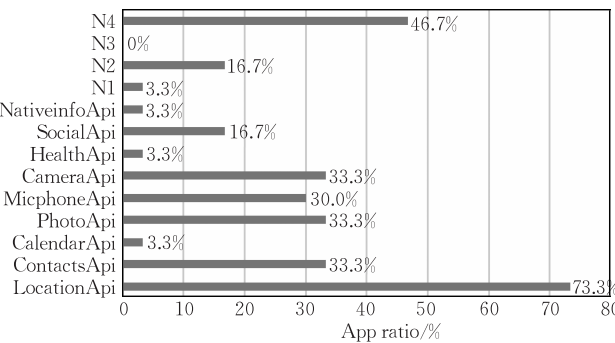
图 13 30 款 iOS 应用程序分析结果
