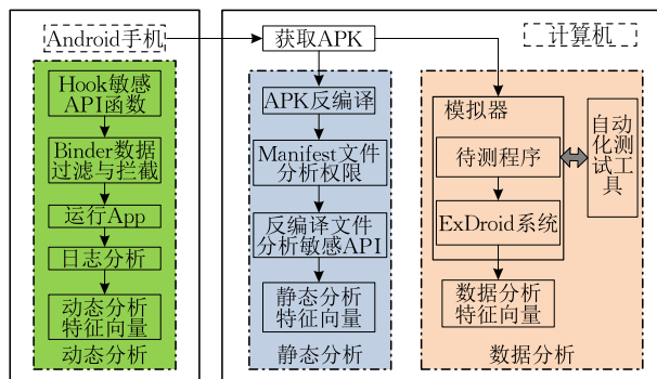
图 2 Android 分析系统实现架构
