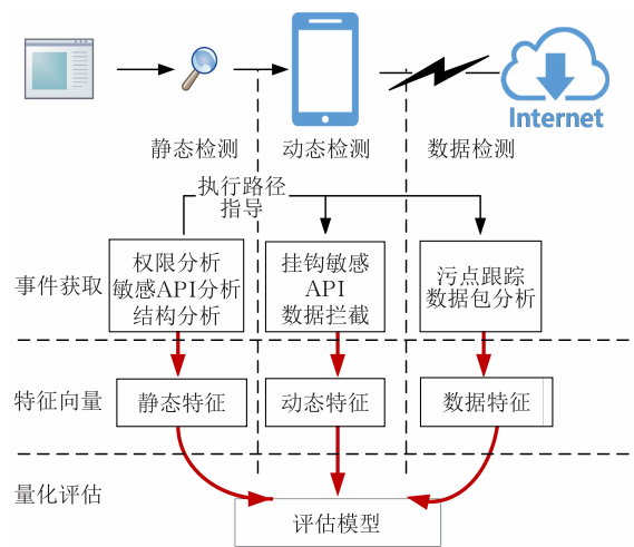
图 1 多维度隐私泄露检测
