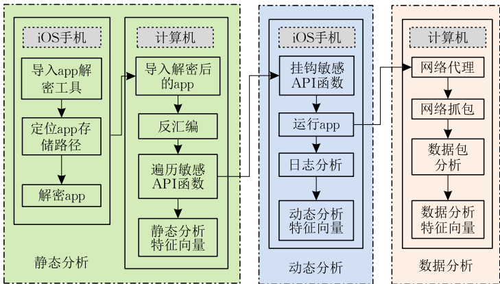
图 5 iOS 分析系统实现框架
