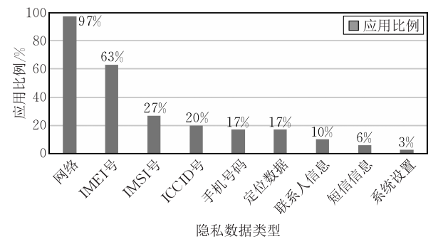
图 12 30 款 Android 应用程序分析结果
