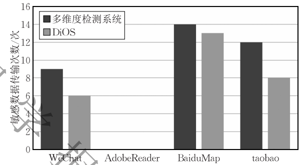
图 10 敏感传输检出次数对比
