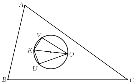
图 2 布洛卡圆定理
