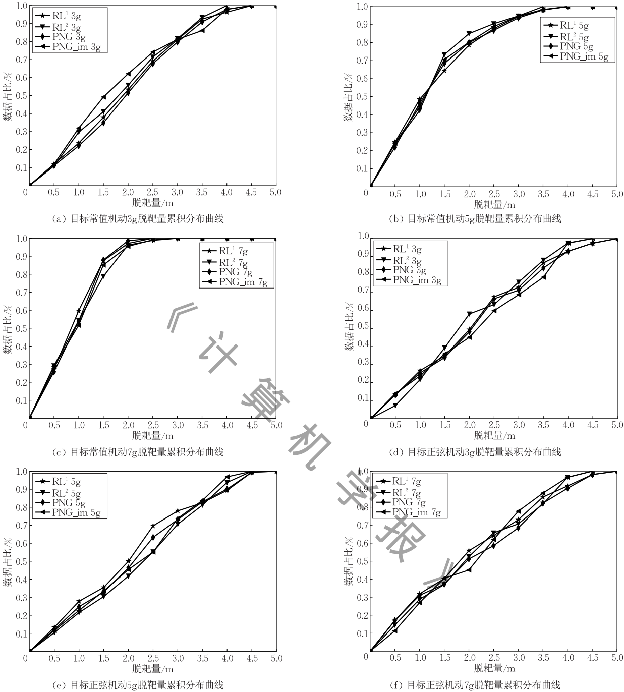
图7 不同机动下脱靶量累积分布曲线
