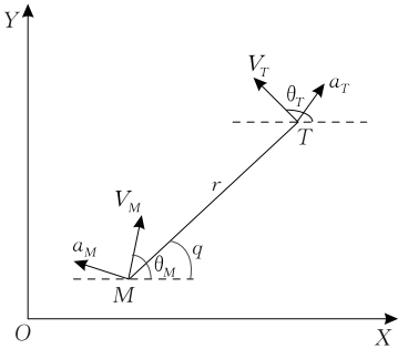
图 1 弹目拦截示意图
