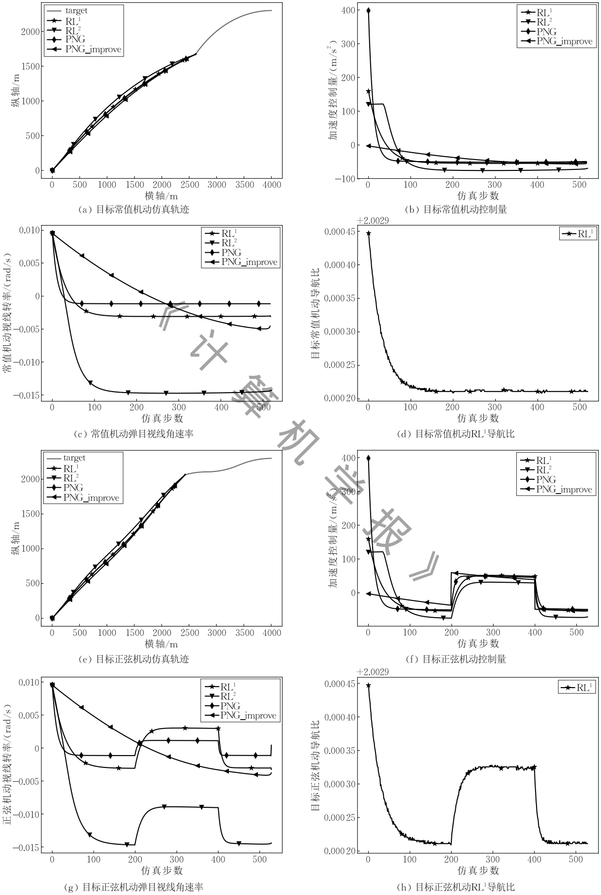
图 6 仿真轨迹、控制量、弹目视线角速度和导航比等对比图
