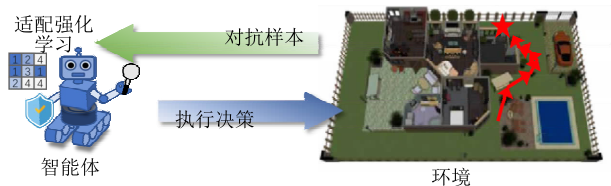
图 11 基于鲁棒学习防御的算法示意图(与传统的防御算法不同,这一类防御方法通常与强化学习算法本身适配,结合了强化学习算法本身的特点)
