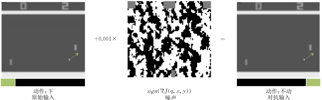
图 3 基于 FGSM 方法生成对抗样本(其通过在输入图像上加入扰动(如中间部分放大后的对抗噪声扰动所示)对智能体的输入空间观测进行攻击, 从而迷惑智能体决策动作(图片下方框为当前动作决策分布) [45] )
