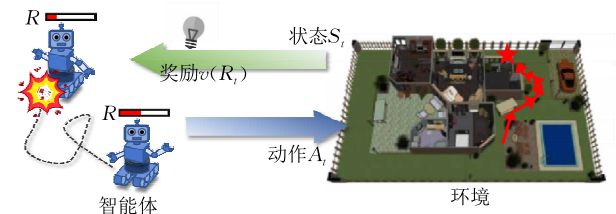
图 5 基于奖励的对攻击算法示意图(对攻击者通过在训练过程中对目标策略的回报奖励加入对抗噪声进行干扰,影响智能体的学习过程,从而达到攻击目的)
