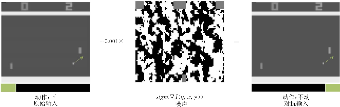
图 3 基于 FGSM 方法生成对抗样本(其通过在输入图像上加入扰动(如中间部分放大的对抗噪声扰动所示)对智能体的输入空间观测进行攻击, 从而迷惑智能体决策动作(图片下方框为当前动作决策分布) [45] )
