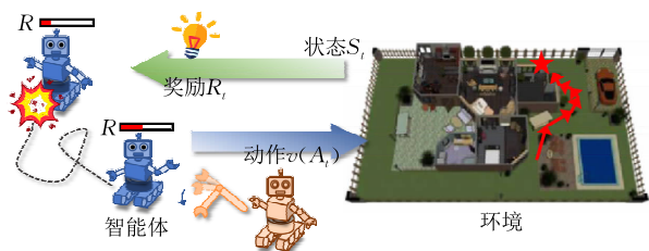
图 6 基于动作的对抗攻击算法示意图(对抗攻击者通过直接扰动智能体输出动作概率或者引入一个具备对抗性策略的智能体进行攻击)
