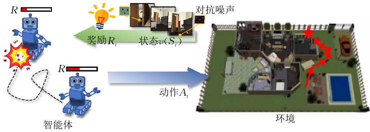
图 2 基于状态的对抗攻击算法示意图(对抗攻击者通过扰动直接动智能体的观测值 s 或在环境中添加对抗噪声来影响智能体的最终决策)
