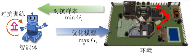
图 8 基于对抗训练防御的算法示意图(对抗训练是在求解一个最小-最大优化问题.在训练过程中,攻击者生成对抗样本给智能体,智能体在具有攻击性环境下优化自身,最终智能体模型会变得更加鲁棒)
