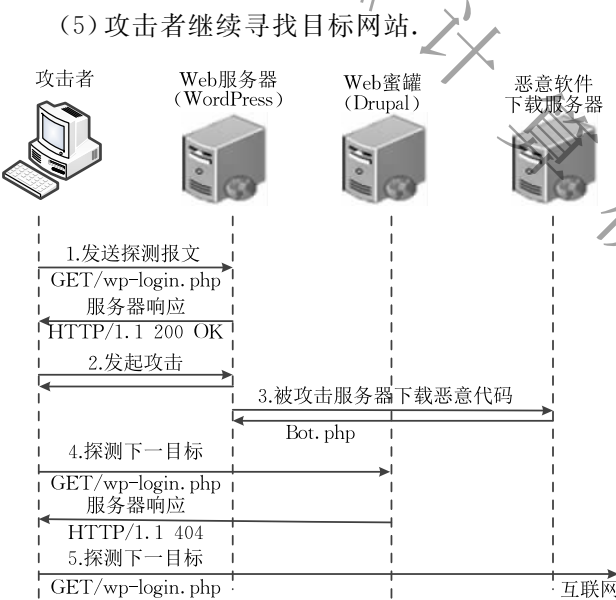
图 1 Web 攻击示意图
