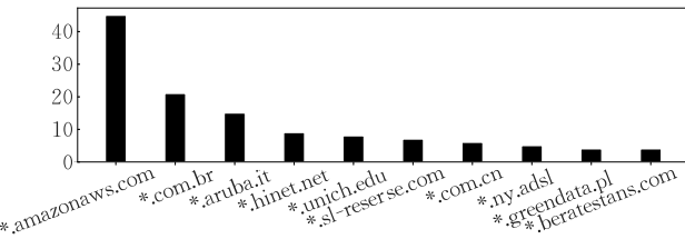
图 8 IP 对应域名统计
