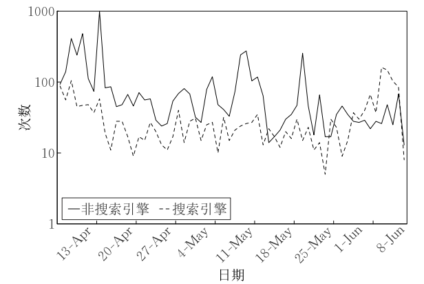
图 6 蜜罐捕获到的 HTTP 流量
