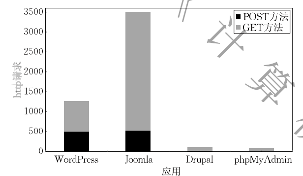
图 9 各个 CMS 吸引的流量
