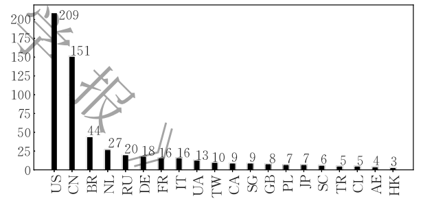
图 7 源 IP 数量前 20 的国家和地区
