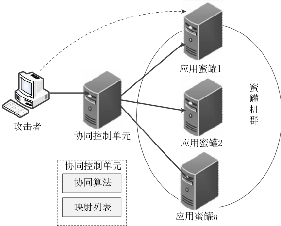
图 3 蜜罐簇概念图
