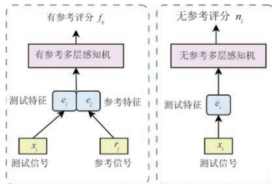
图 10 CORN 算法框架 [136]
