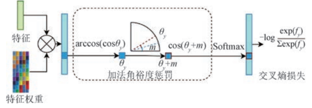
图 11 利用 ArcFace 损失训练 DCNN 网络 [137]
