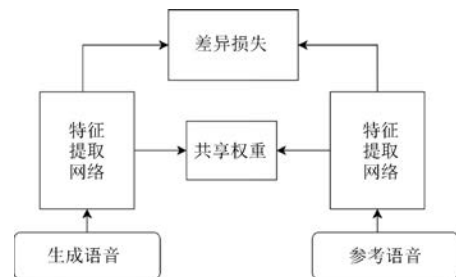
图 19 语音评测的双流架构 [142]
