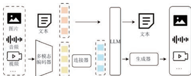
图 17 MLLM 架构 [217]
