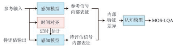
图 8 POLQA 算法框架 [118]
