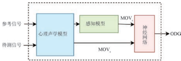
图 7 PEAQ 算法框架 [117]
