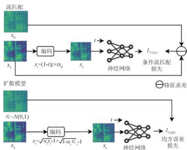
图2 扩散与流匹配 TTS 对比
