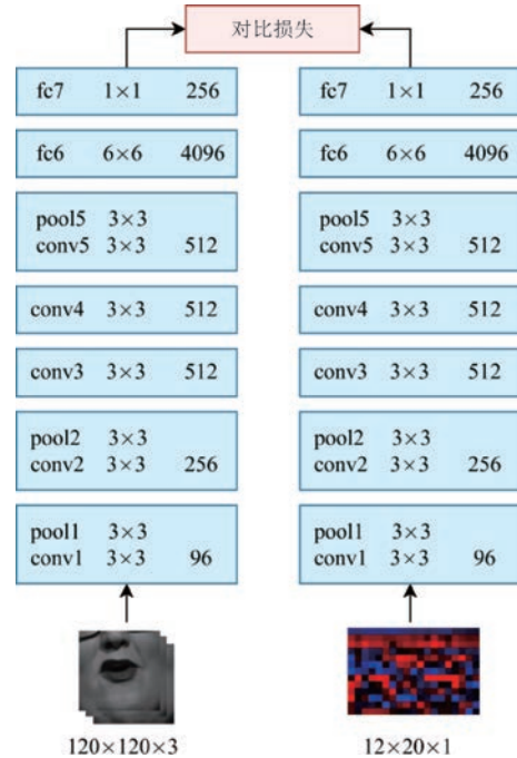
图 12 SyncNet 架构 [142]
