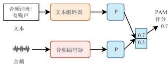
图 9 PAM 算法框架 [135]
