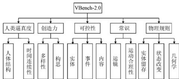
图 13 VBench-2.0 的评测维度
