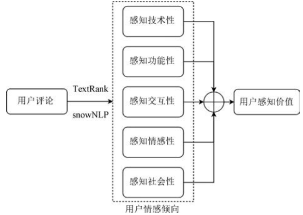
图 15 用户感知视角下数字人评测模型 [186]
