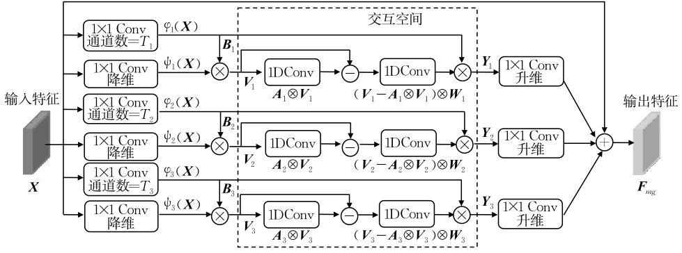
图 3 多重图卷积结构示意图
