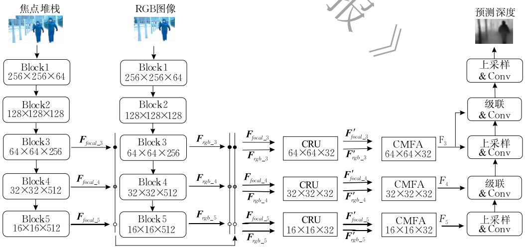
图 1 基于多模态信息的深度估计网络示意图(此结构由编码器和解码器两部分组成,编码器部分每一支路包括 5 个卷积块和 3 个 CRU 模块,每一支路的第 3,4,5 层特征将通过一个 CRU 单元;解码器部分包括 CMFA 模块和多个级联、卷积、上采样模块)
