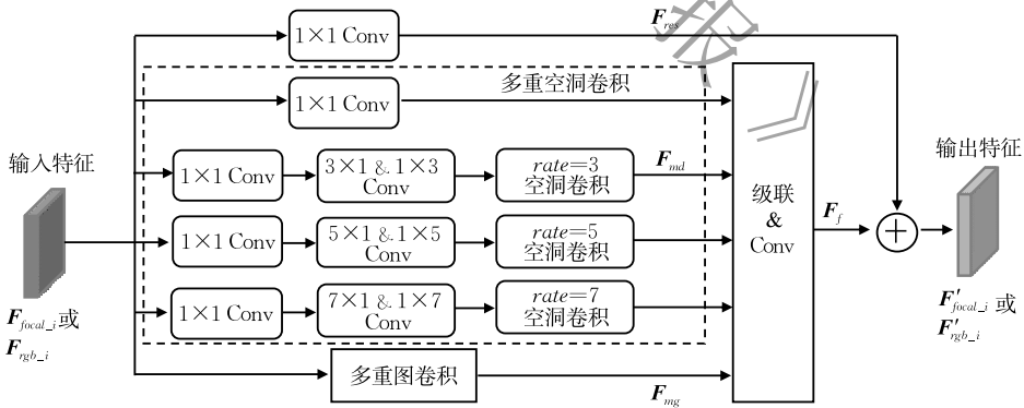
图 2 上下文推理单元(CRU)结构示意图
