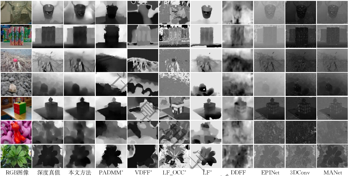
图 8 本文方法和其他方法在 DUT-LFDD 数据集上的预测深度图
