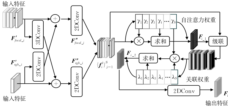
图 4 注意力引导的跨模态融合模块(CMFA)结构示意图
