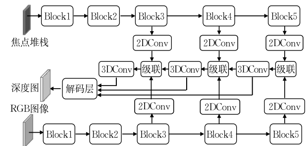
图 5 基线网络模型示意图
