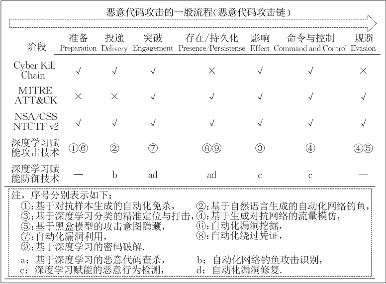
图 1 基于恶意代码攻击链的赋能技术分类
