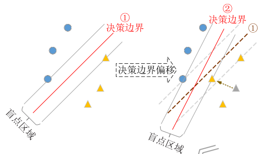
图 10 模型决策边界示意图
