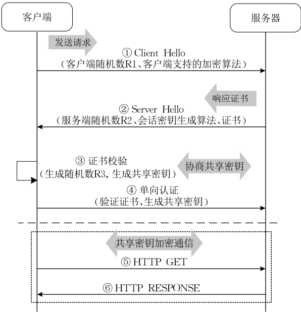
图 9 HTTPS 通信流程
