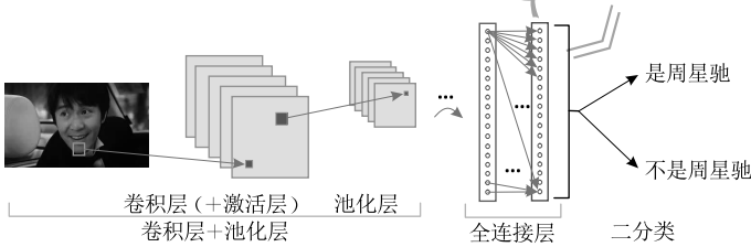
图 4 基于深度神经网络的特定目标识别示意图
