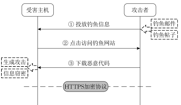
图 8 基于 HTTPS 的钓鱼攻击流程
