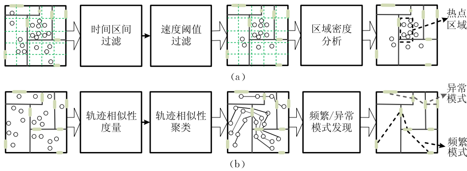
图 13 室内空间热点区域和移动模式分析示意
