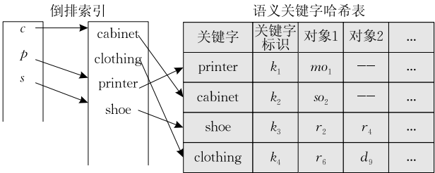
图 12 语义关键词哈希表及其倒排索引结构图示例
