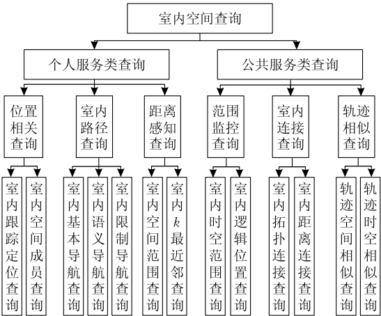
图 3 室内空间查询分类示意图
