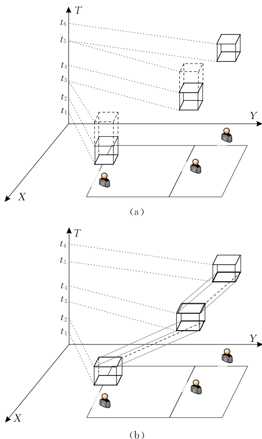
图 4 室内移动对象轨迹插值示例
