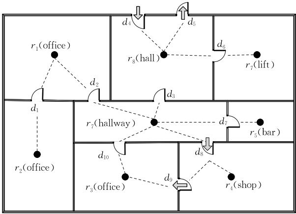
图 6 室内空间布局示例
