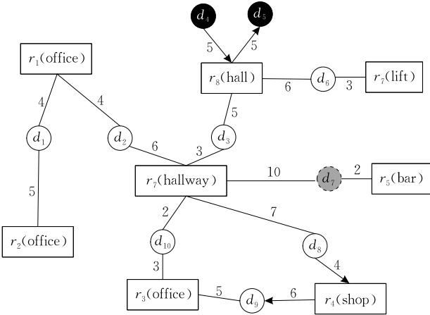
(a) 有向连通图模型
