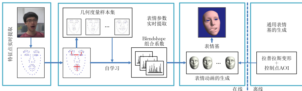
图 1 面部动画生成算法框图
