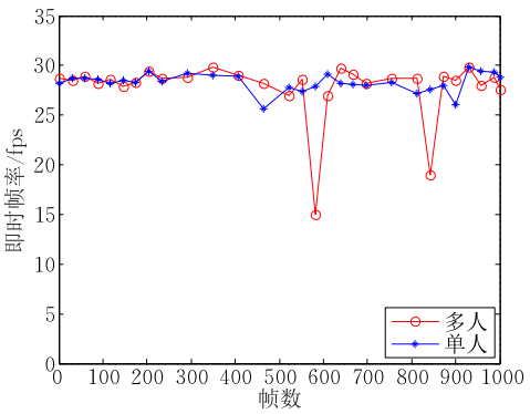
图 16 帧数与即时帧率之间的关系
