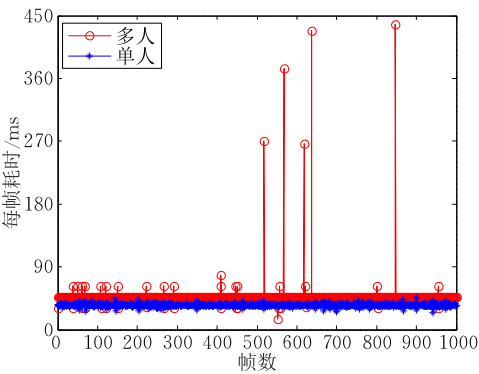
图 15 帧数与每帧耗时之间的关系
