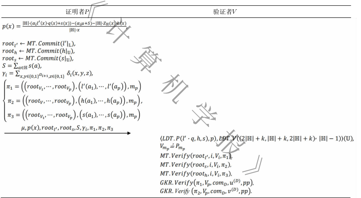
图 3 非交互零知识可验证多项式委托
