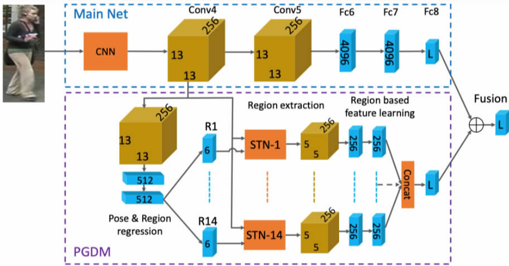
图 12 PGDM 方法的模型结构图
