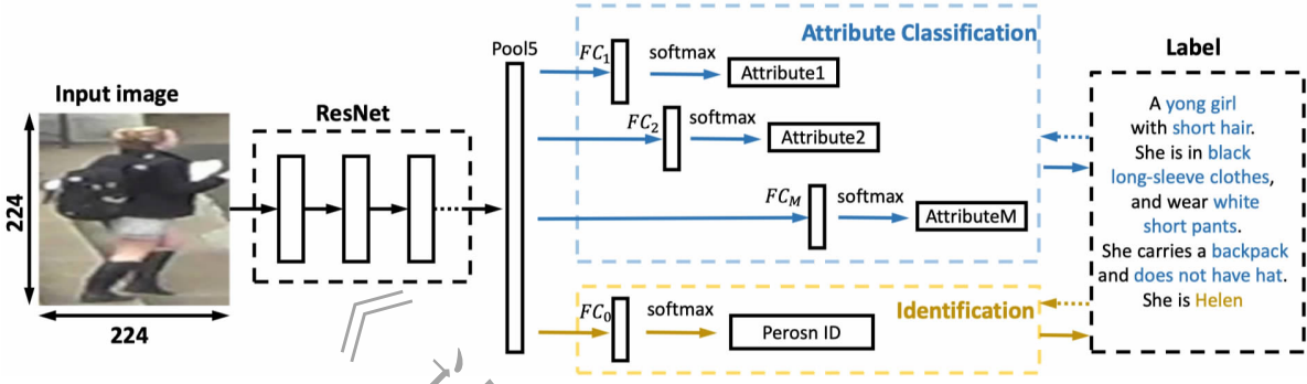
图 31 APR 方法的模型结构图
