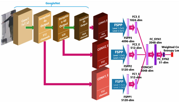
图 7 WPAL 方法的模型结构图
