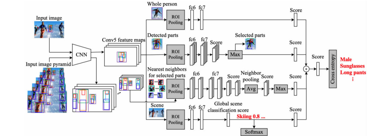
图 29 DHC 方法的模型结构图
