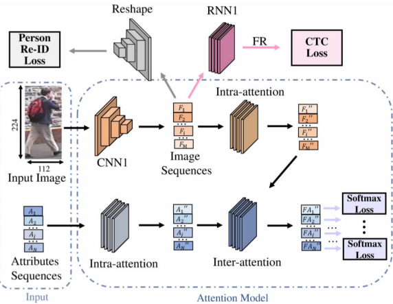
图 27 SCRL 方法的模型结构图
