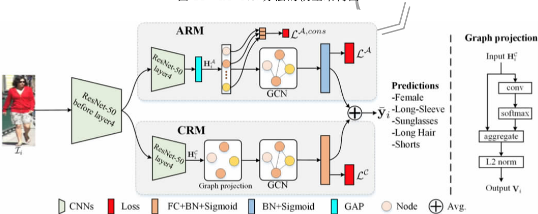
图 22 JLAC 方法的模型结构图
