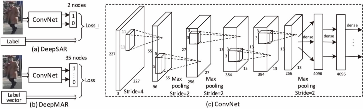
图 6 DeepMAR 方法的模型结构图
