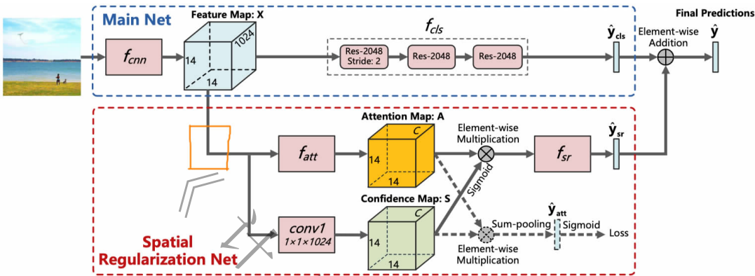
图 30 SRN 方法的模型结构图
