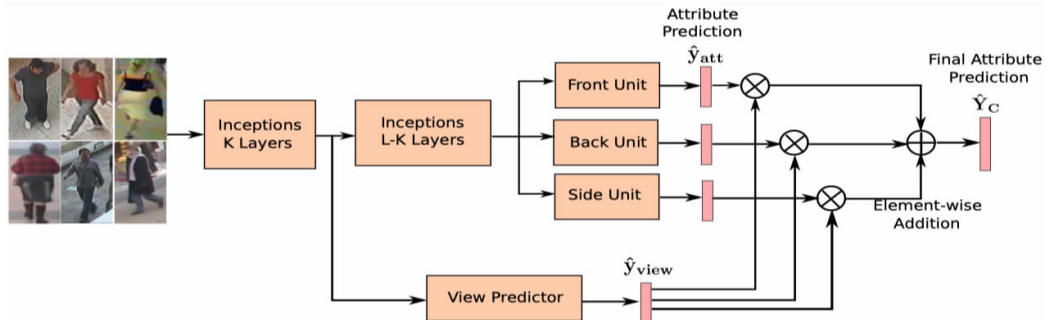
图 8 VeSPA 方法的模型结构图
