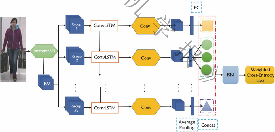
图 15 RC&RA 方法的模型结构图
