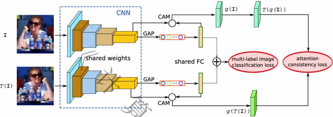
图 19 VAC 方法的模型结构图
