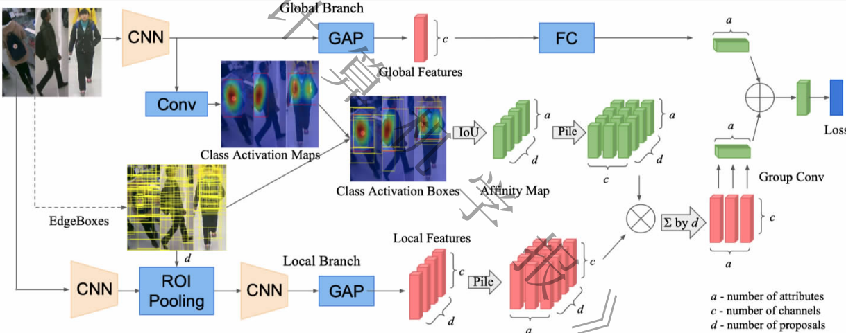
图 11 LGNet 方法的模型结构图
