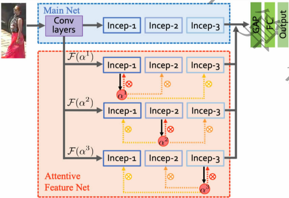
图 9 HPNet 方法的模型结构图
