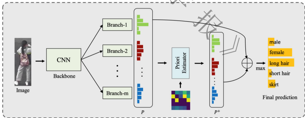
图 18 AAP 方法的模型结构图
