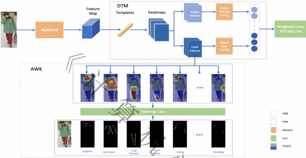
图 25 DTM 方法的模型结构图
