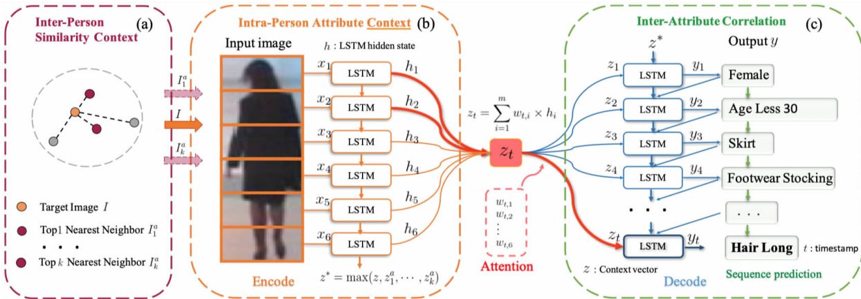
图 10 JRL 方法的模型结构图
