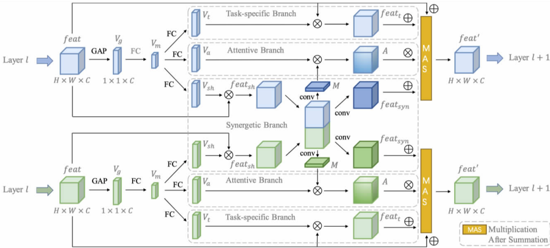
图 24 CAS 方法的模型结构图
