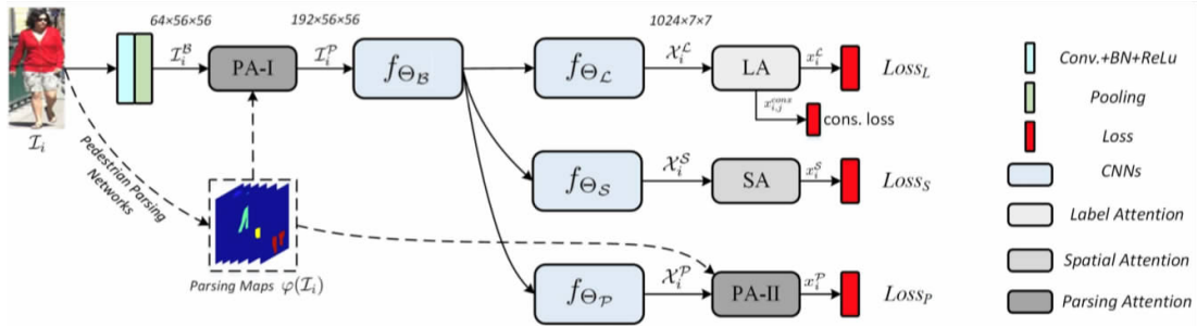
图 26 JLPLS-PAA 方法的模型结构图
