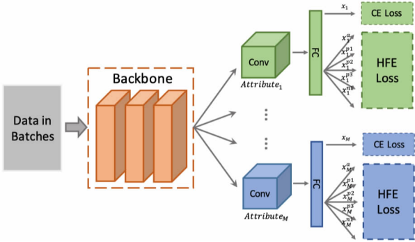
图 32 HFE 方法的模型结构图
