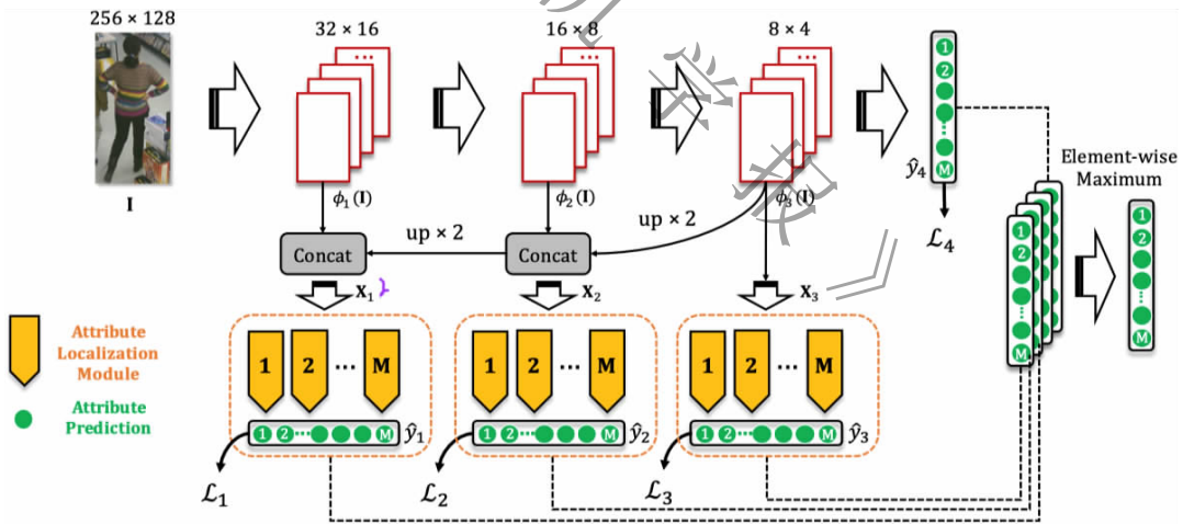
图 20 ALM 方法的模型结构图
