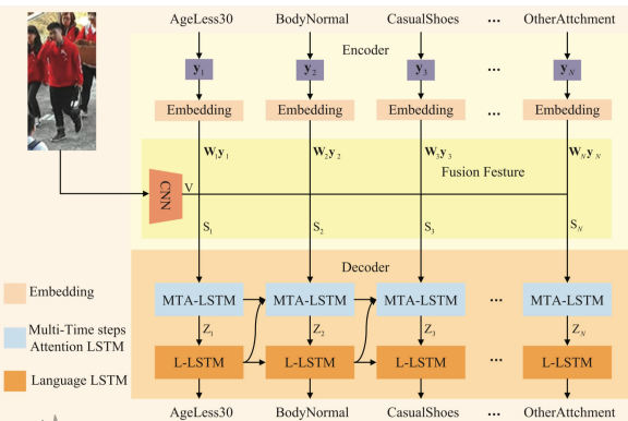
图 28 MTANet 方法的模型结构图
