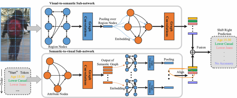
图 16 VSGR 方法的模型结构图
