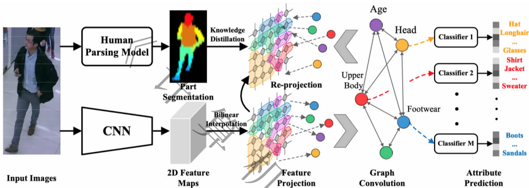
图 17 GRKD 方法的模型结构图
