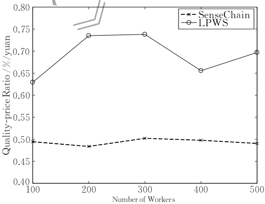
图 8 质价比较
