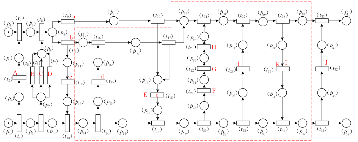
图 6 目标模型控制流和数据流的融合网
