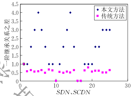
(c) 存在沉默变迁情况下的 SDN 和 SCDN 的一阶继承关系之差
