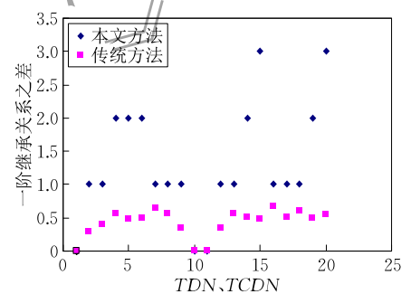
(d) 存在沉默变迁情况下的 TDN 和 TCDN 的一阶继承关系之差
