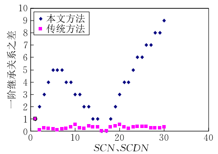
(a) 存在沉默变迁情况下的 SCN 和 SCDN 的一阶继承关系之差
