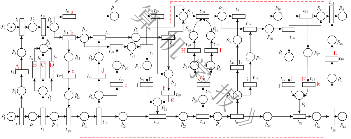
图 5 源模型控制流和数据流的融合网
