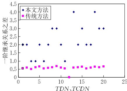
(d) 无沉默变迁情况下的TDN和TCDN的一阶继承关系之差
