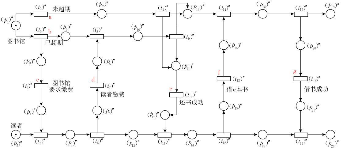
图 4 目标模型数据流网
