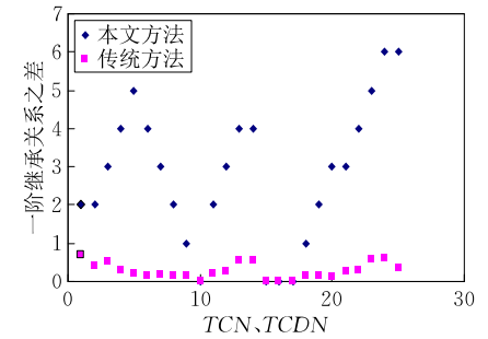
(b) 存在沉默变迁情况下的 TCN 和 TCDN 的一阶继承关系之差
