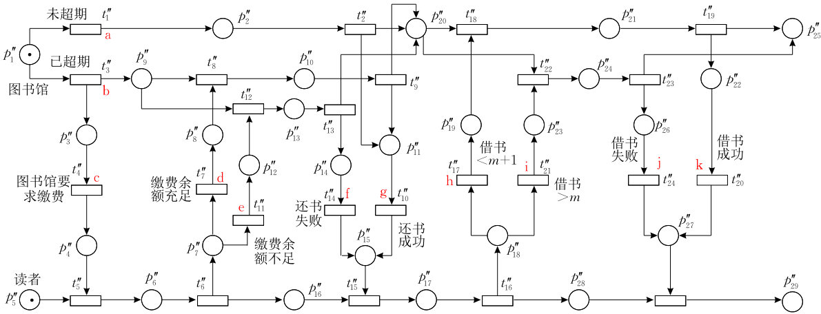
图 3 源模型数据流网
