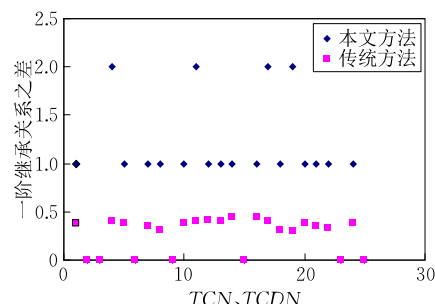
(b) 无沉默变迁情况下的TCN和TCDN的一阶继承关系之差
