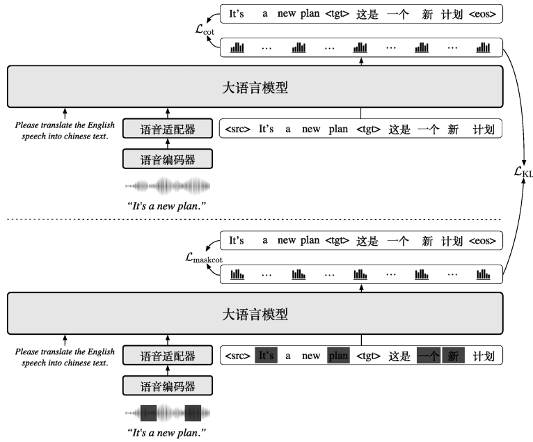
图 2 模型结构与训练方法示意图
