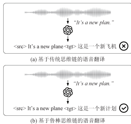
图 1 基于鲁棒思维链的语音翻译示意图
