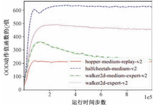
图 9 OOD 动作值函数 Q(s^{in}, a^{ood}) 的 Q 值估计
