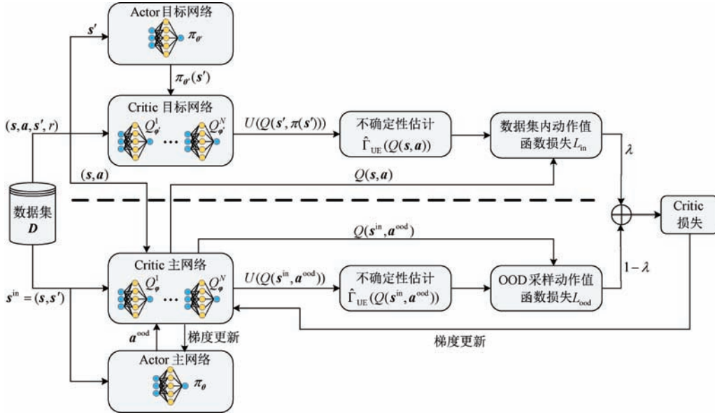
图 1 ODACUE 的整体框架
